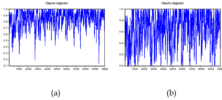
Şekil 9. Durum (iii) \alpha = 0,3 ve \omega = 0,3 hipotez testi sonuçları
