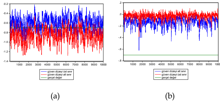
Şekil 2. Durum (i) \omega = 0,9 ve \alpha = 0,3 güven düzeyi sonuçları
