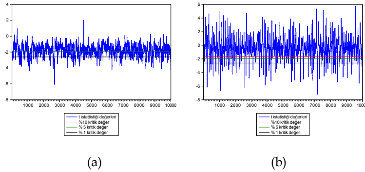
Şekil 4. Durum (ii) \alpha = 0,9 ve \omega = 0,9 \hat{t} testi sonuçları
