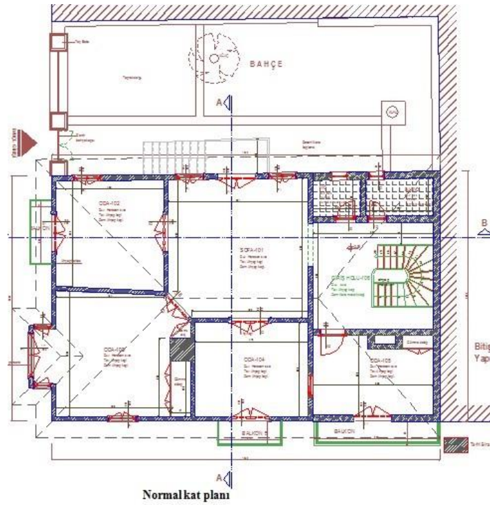
Şekil 111: K-2 Giriş Kat Planı
