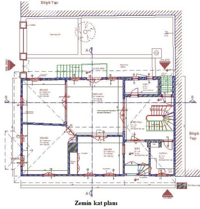
Şekil 110: K-2 Bodrum Kat Planı
