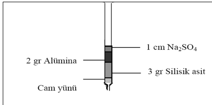
Şekil 3.4. Temizleme kolonu
