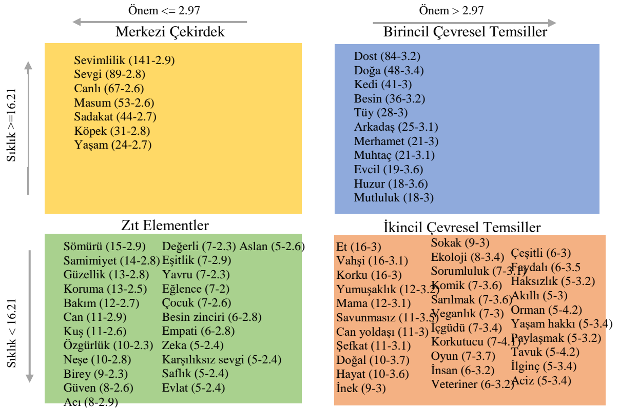
Şekil 14. Türçülük düzeyi yüksek olan grubun hayvan temsiline dair prototip analiz sonuçları
