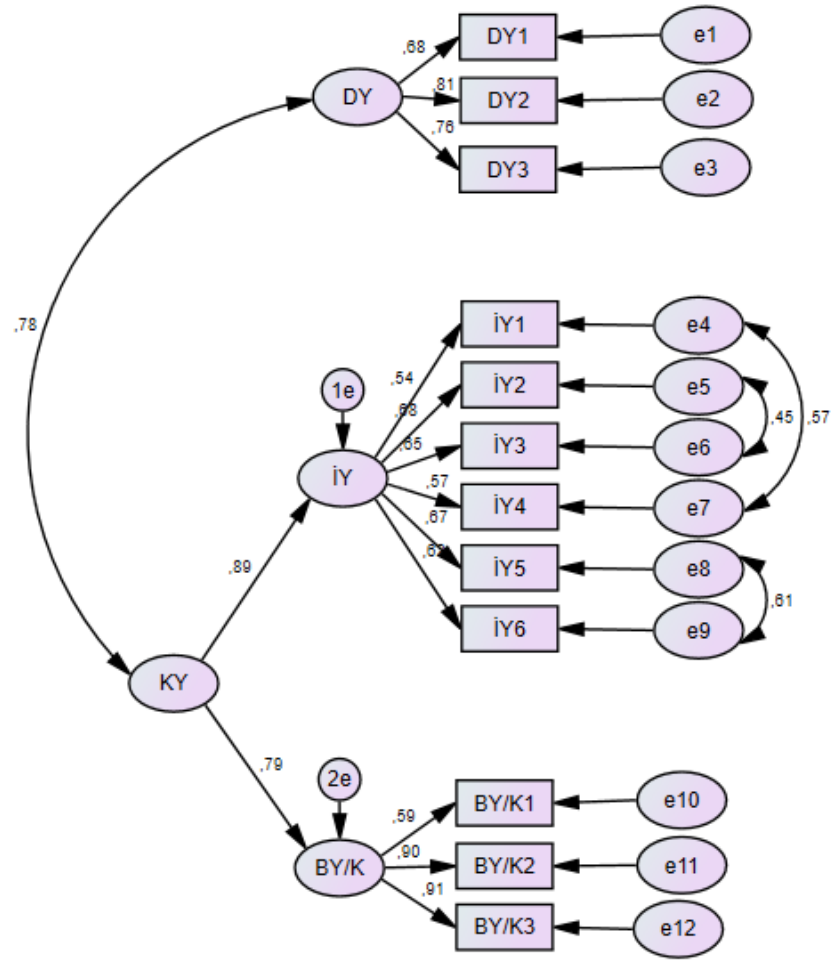
Şekil 6. ÇYÖ'nün DFA modeli
