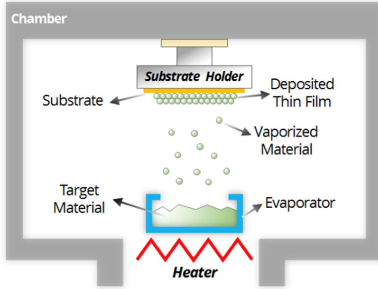
Şekil 2.5. Termal buharlaştırma film biriktirme yönteminin şematik gösterimi (Park 2016)
