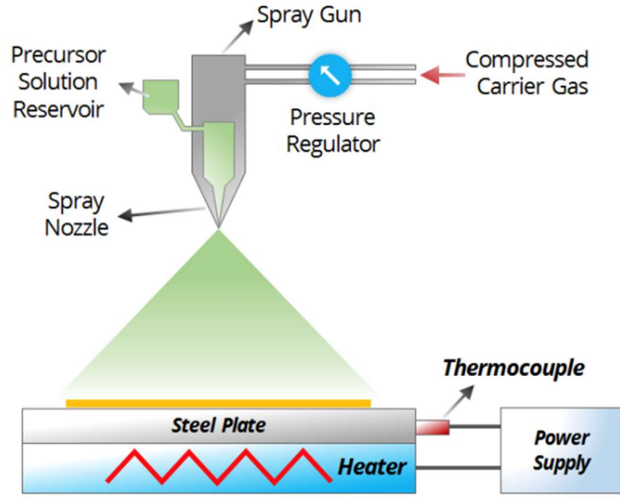
Şekil 2.3. Sprey-piroliz yönteminin şematik gösterimi (Park 2016).
