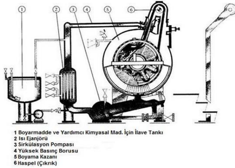
Şekil 3. 8. Jet boyama makinesi (Dağkurs ve İşeri, 2018)
