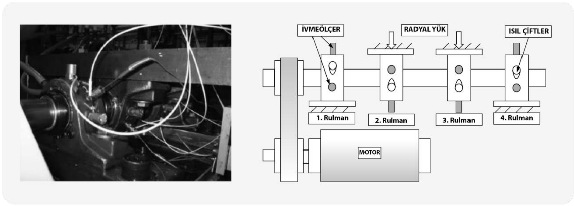
Şekil 3.1. NASA rulman veri seti test mekanizması yerleşimi (J. Lee, H. ve arkadaşlarının 2007’de yaptıkları çalışmadan değiştirilerek alınmıştır.)
