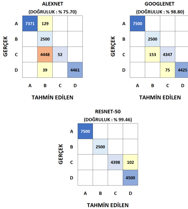
Şekil 4.4. Eğitim modellerinin test verileriyle oluşturduğu karışıklık matrisi (A: İç yatak arızası, B: Normal durum, C: Dış yatak 1. rulman, D: Dış yatak 3. rulman)
