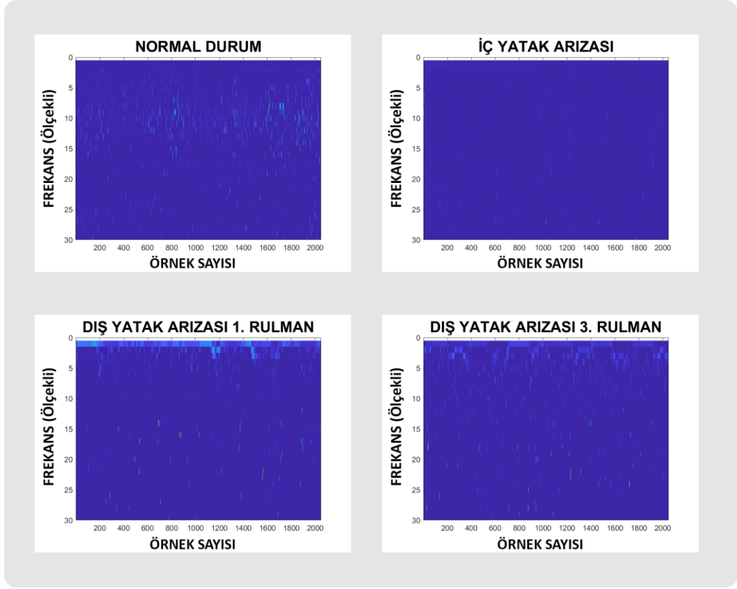
Şekil 3.8. NASA rulman veri seti ile Hilbert Huang dönüşümü
