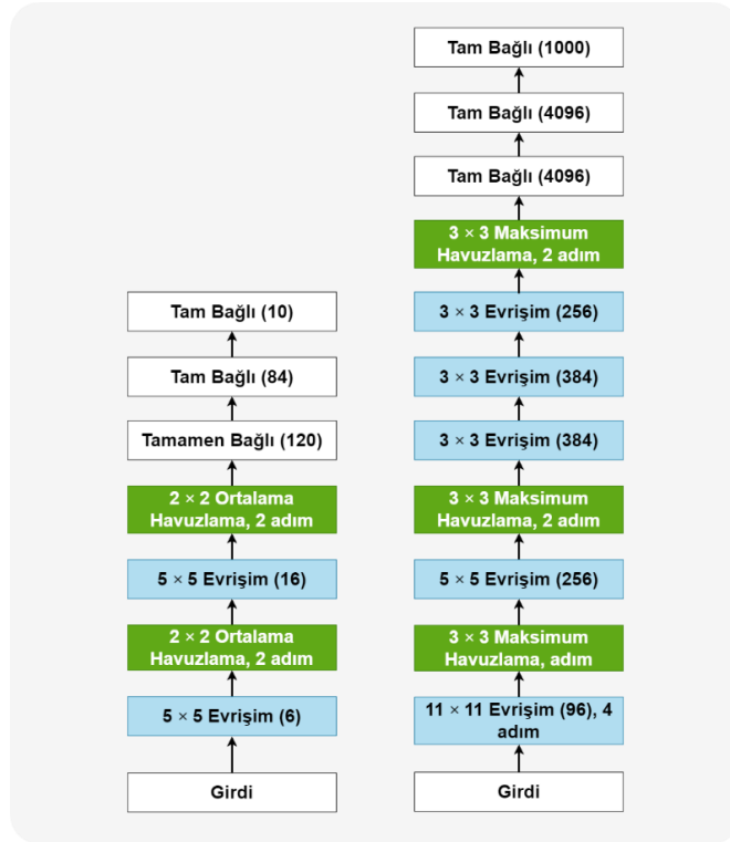
Şekil 2.9. AlexNet(sağ) ve LeNet(sol) mimarileri (Zhang, A. ve ark. 2021)’nın çalışmalarından değiştirilerek alınmıştır.)
