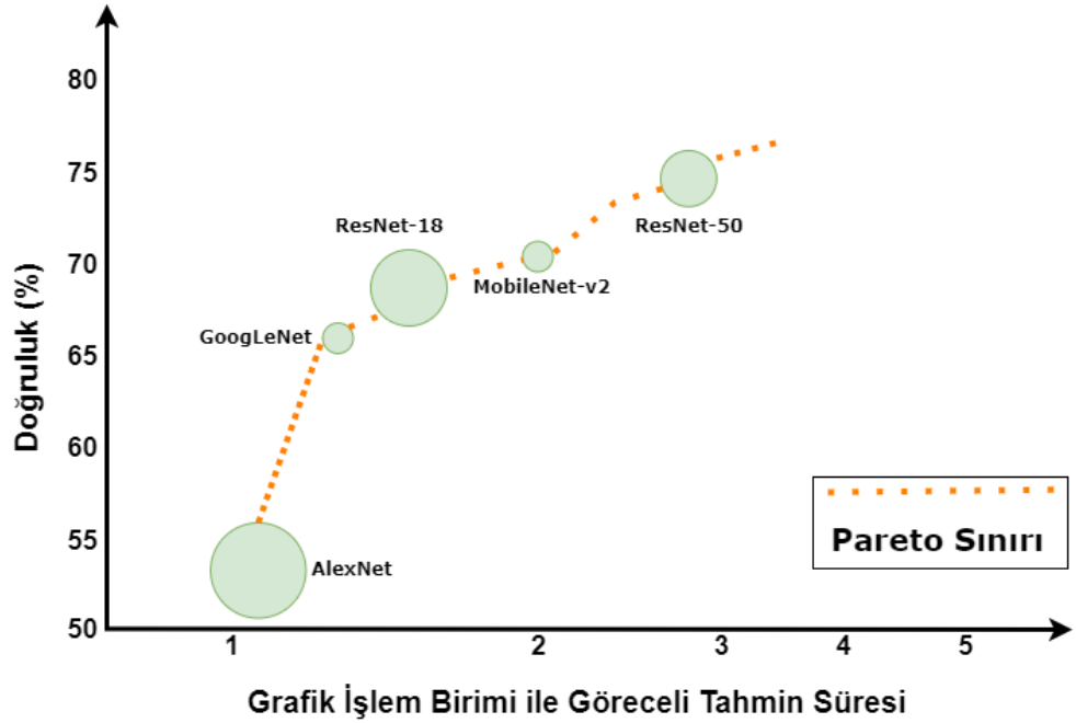
Şekil 2.6. Önceden eğitilmiş ađların karşılaştırılması (Pan, S. J., ve Yang, Q.’nin 2010’daki çalışmasından değiştirilerek alınmıştır.)
