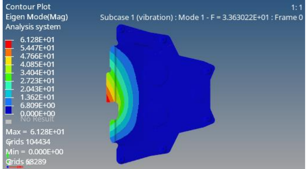
Şekil 4.14. Model 7 Daire Tam (DT) Modal Analiz Sonucu
