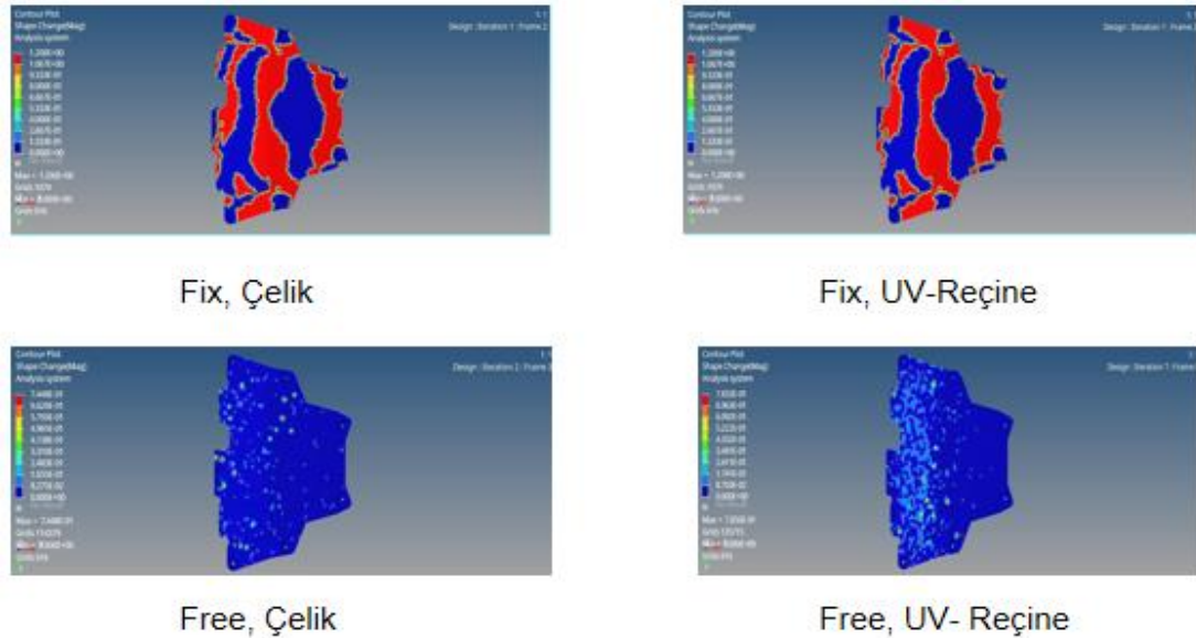
Şekil 4.23. 0.575 ölçeğindeki mesnetli ve serbest haldeki modellerin topografya sonuçları
