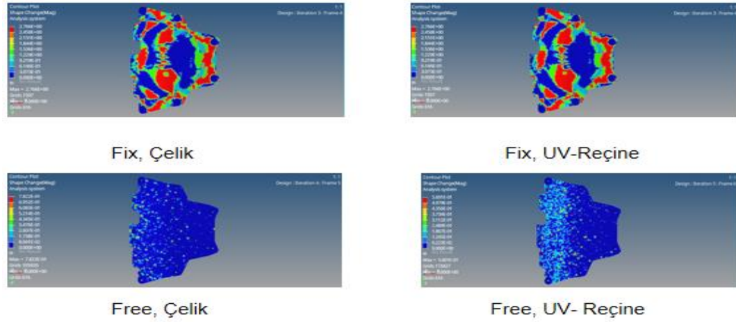
Şekil 4.22. 0.7875 ölçeğindeki mesnetli ve serbest haldeki modellerin topografya sonuçları
