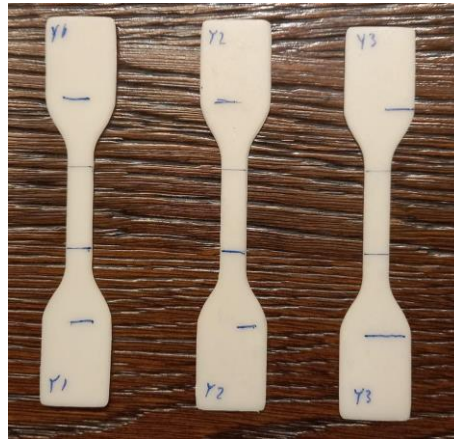
Şekil 3.8. Çekme numunelerin hazırlanmış gösterimi
