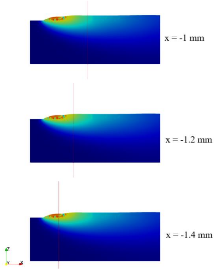
Şekil 3.12. Sıcaklık değişimini incelemek için x ekseninde ölçüm alınan kesitler
