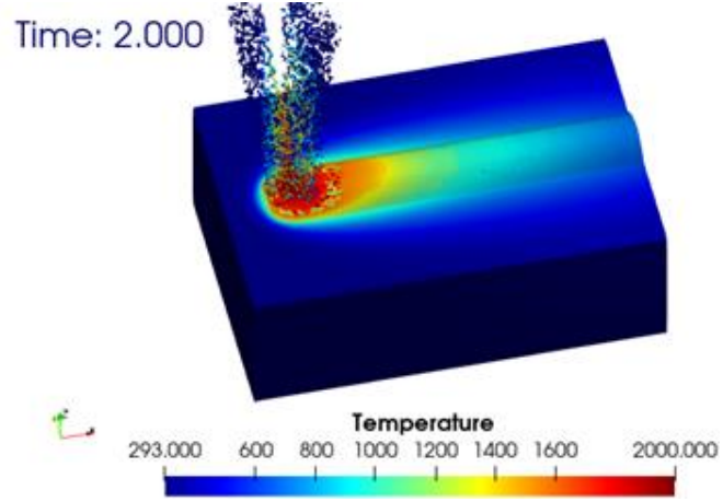
Őekil 3.11. 3 nozuldan toz parçacıklarının püskürtülmesi
