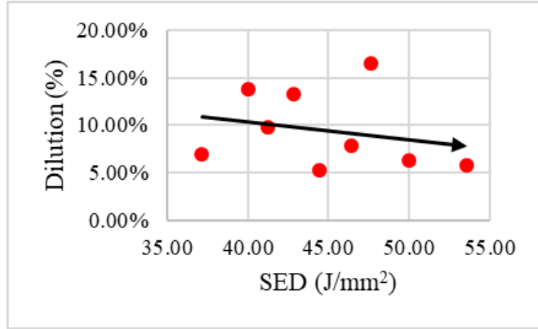
Şekil 4.9. SED'in dilution üzerindeki etkileri
