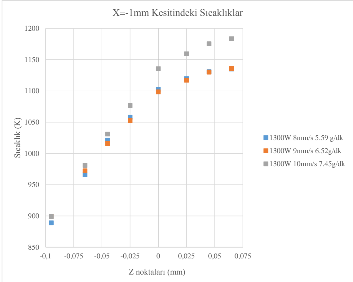
Şekil 4.21. x = -1\text{mm} kesitindeki 1300W için sıcaklık dağılımı
