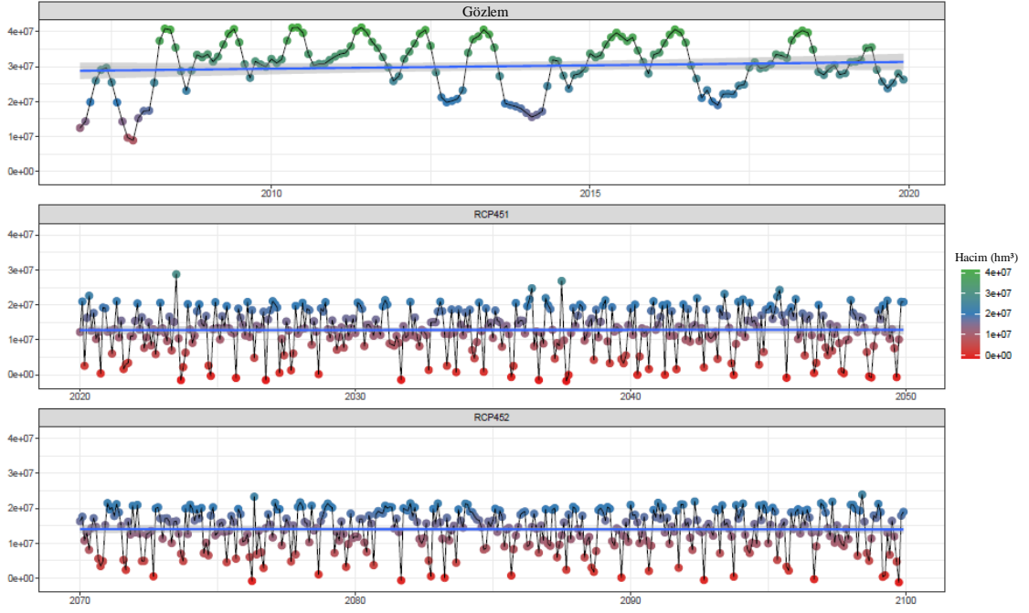
Şekil 28. Barajdaki hacim miktarının RCP 4.5 senaryosu temelinde zamansal değişim grafiği
