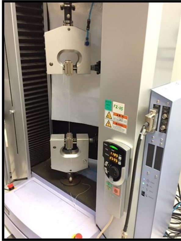
řekil 3.26. Mukavemet lm cihazı
