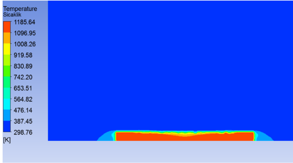
Şekil 4.6. Parça orta düzleminde sıcaklık dağılımı (H=275 mm, t=1 s)
