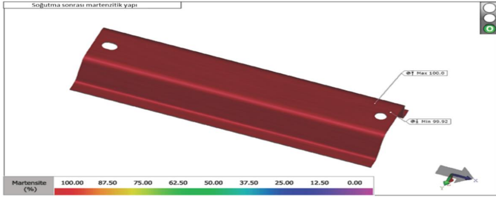
Şekil 3.7. %100 martenzit yapıya ulaşması analizi (Autoform thermosolver)
