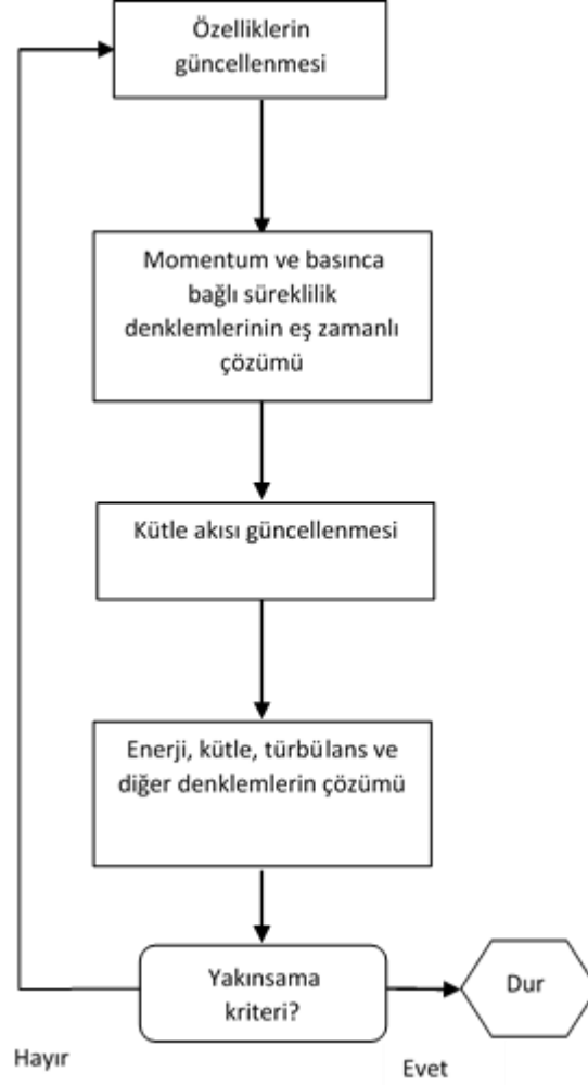
Şekil 3.22. Basınca bağı eş zamanlı çözüm metoduna ait akış diyagramı (Ying 2017)
