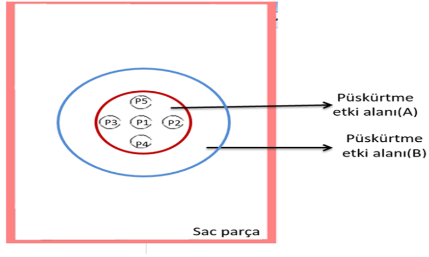
Şekil 3.19. Sprey soğutma için tanımlanmış noktaların konumu
