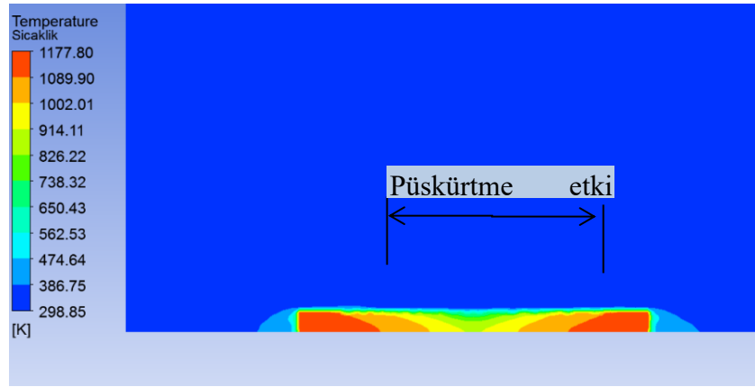
Şekil 4.9. Parça orta düzleminde sıcaklık dağılımı (H=275 mm, t ~ 5 s)
