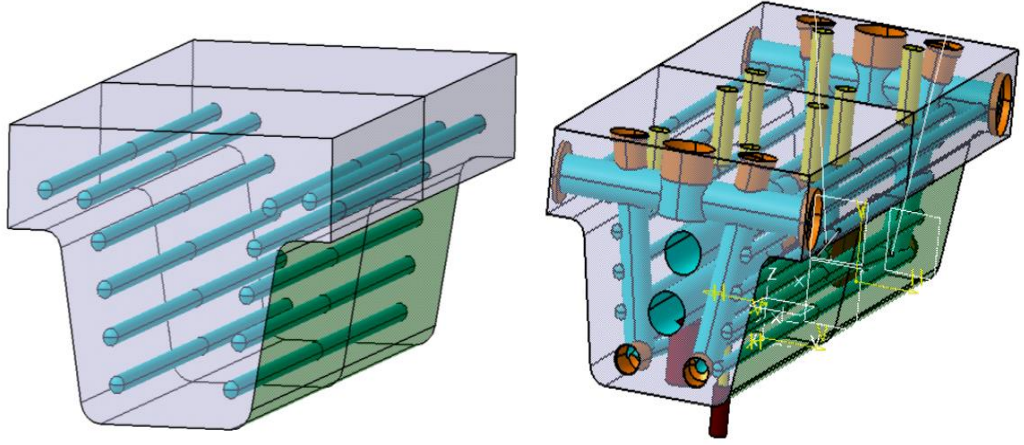
Şekil 3.14. Üst çelik grubu (Catia-V5)
