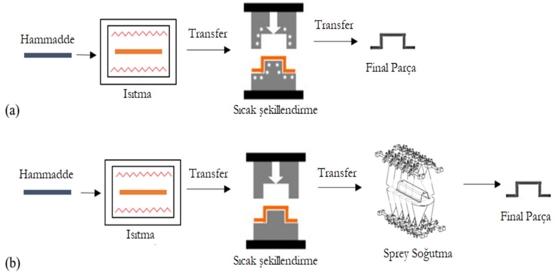
Şekil 2.1. (a) Sıcak şekillendirme işleminin ve (b) Çok ağızlı hibrit su verme sıcak şekillendirme işlemlerinin aşamaları. (Park ve ark. 2015 – jenerik gösterim)
