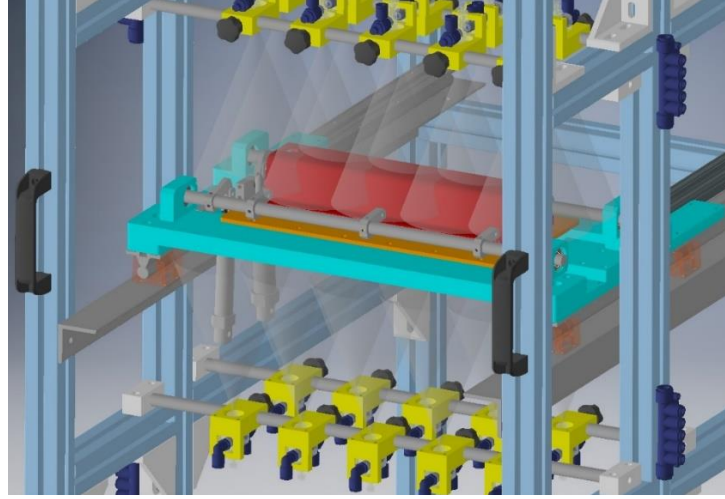
Şekil 3.33. Sprey soğutma sistemi nozul gösterimi-2
