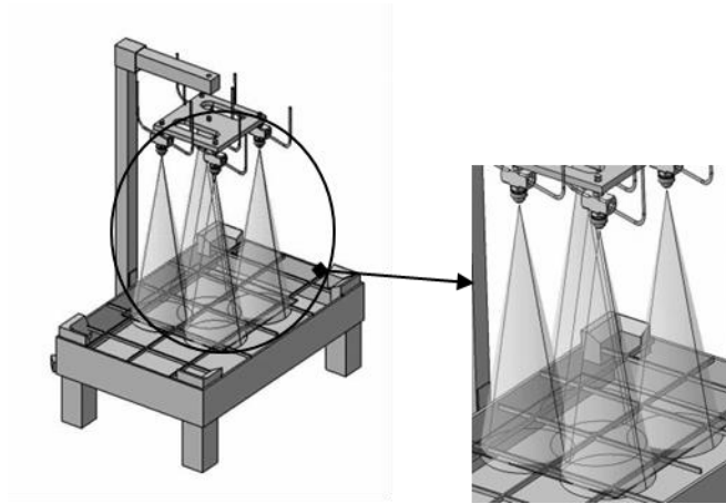
Şekil 3.29. Hibrit su verme için geliştirilmiş püskürtme nozulu fikstürü (Catia-V5)
