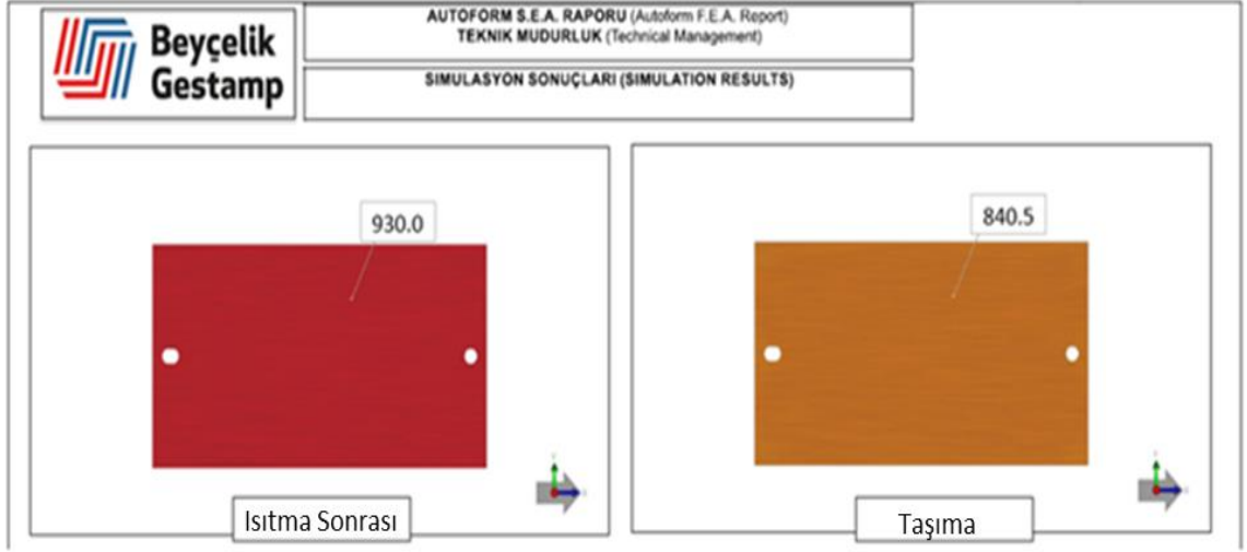
Şekil 3.5. Sacın fırından prese taşındığında sıcaklık değişimi (Autoform thermosolver)
