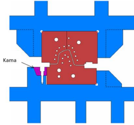
Şekil 3.10. Kamaların yerleşimi (Kalıp standartları jenerik gösterim)
