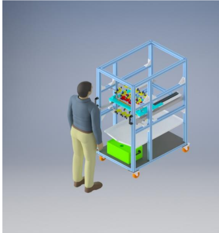
Şekil 3.31. Sprey soğutma sistemi tasarımı-2
