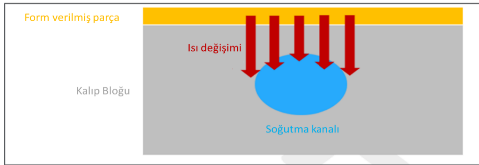
Şekil 2.10. Kalıp içerisinde ısı akışı ve soğutma kanalı tasarımı (Fernandez ve ark. 2019)
