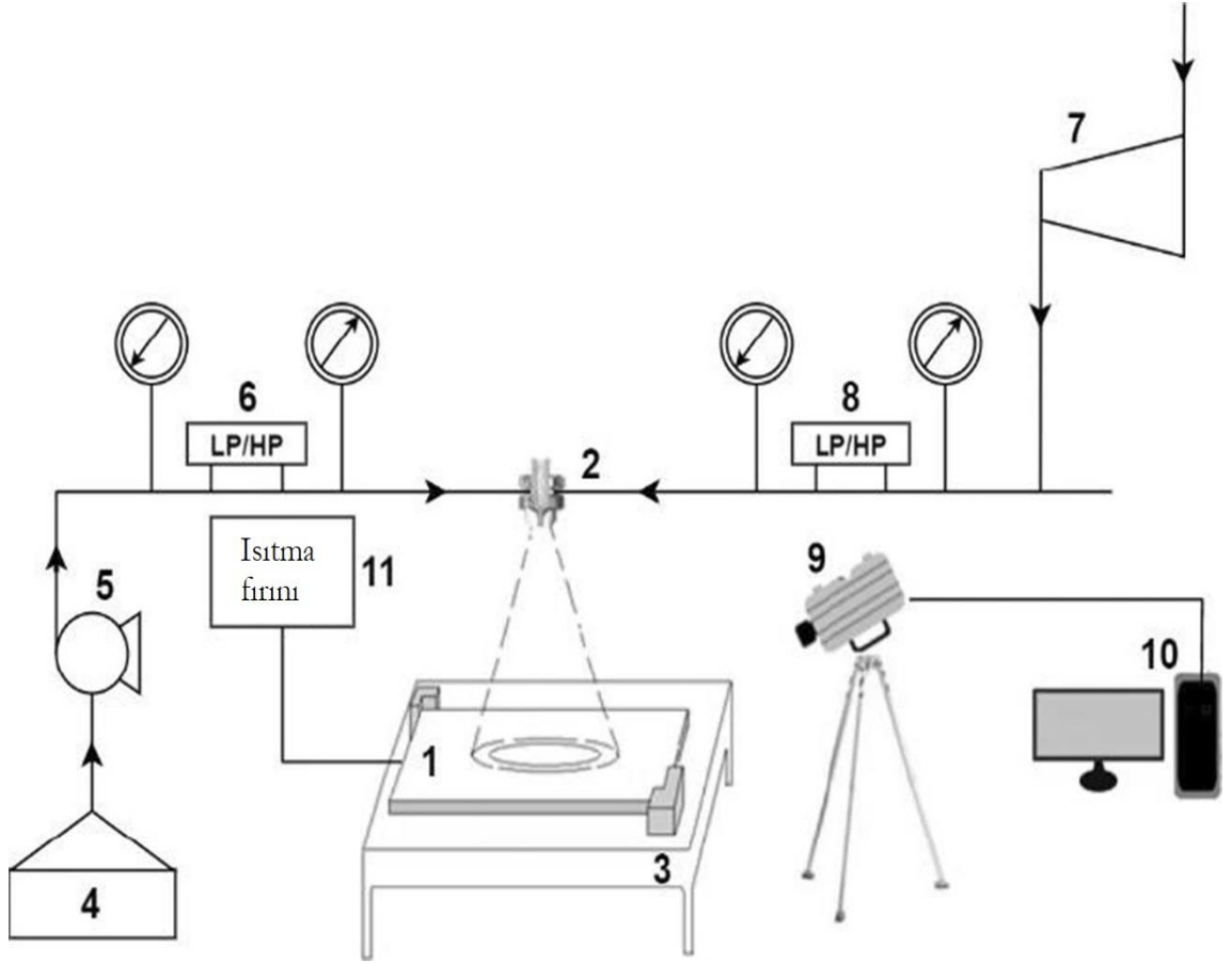
Şekil 3.23. Deneylerde kullanılan püskürtme aparatı ve kızılötesi termal kameranın jenerik görseli (Ying 2017)
