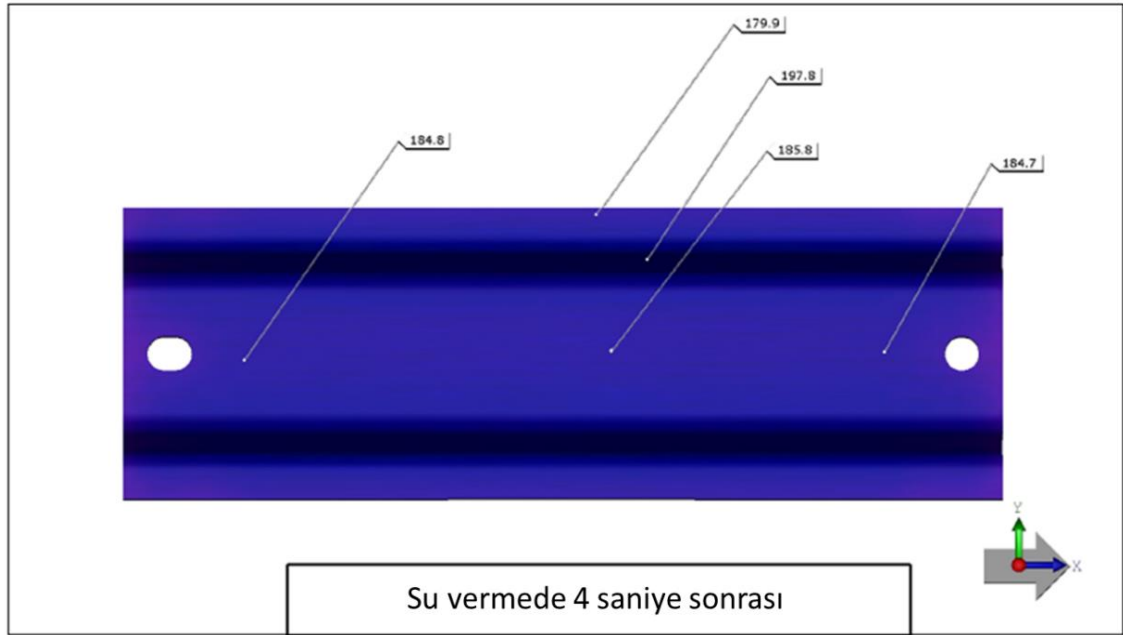
Şekil 3.6. Parçaya 4 sn su verilip kalıp içerisinde tavlama işleminin tamamlanması (Autoform thermosolver)
