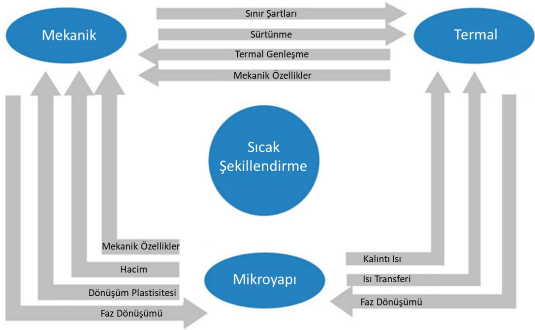
Şekil 3.1. Sıcak şekillendirme simülasyon parametreleri ve etkileşimleri (Shuo-shuo ve ark. 2021)
