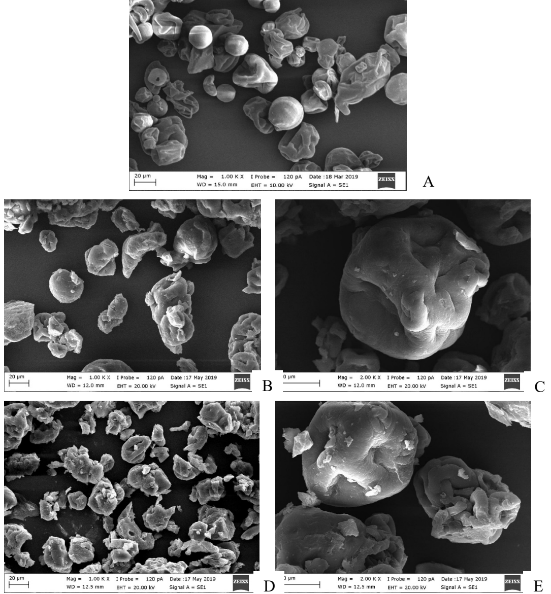
Şekil 4.9. Yüklü ve yüklü olmayan Spirulina ’ların yüzeylerinin SEM görüntüleri A) Boş Spirulina B) ve D) Spirulina /hidroalkolik ve Spirulina /sulu ekstraktları (1000x büyütme) C) ve E) Spirulina /hidroalkolik ve Spirulina /sulu ekstraktları (2000x büyütme)
