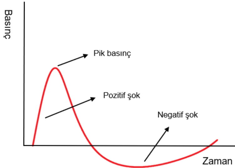
Şekil-3: Tipik bir radial şok dalga paterni
