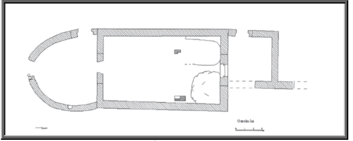
a- Gazelin İni Çiftlik Villası Plan
