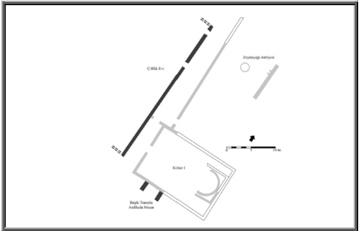
b- Özköy Çiftlik Villası Plan
