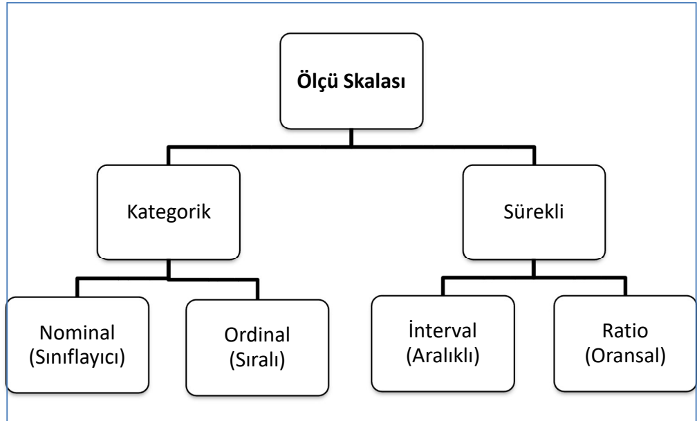
Şekil 1: Veri Türleri
