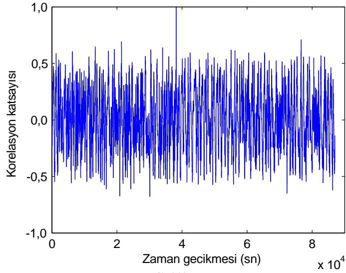
Şekil 5: İşlek bir caddede çekilen 10 dakikalık videodan (Video 2) kestirilen ENF sinyali ile referans ENF sinyalinin çapraz korelasyonu-Maksimum korelasyon katsayısı referans sinyalin 37617. saniyesinde bulunmuştur
