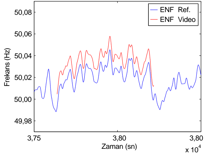
Şekil 6: İşlek bir caddede çekilen 10 dakikalık videodan (Video 2) kestirilen ENF sinyali ile referans ENF sinyalinin korelasyon katsayısının en yüksek bulunduğu noktada (37617. saniye) üst üste çizdirilmesi
