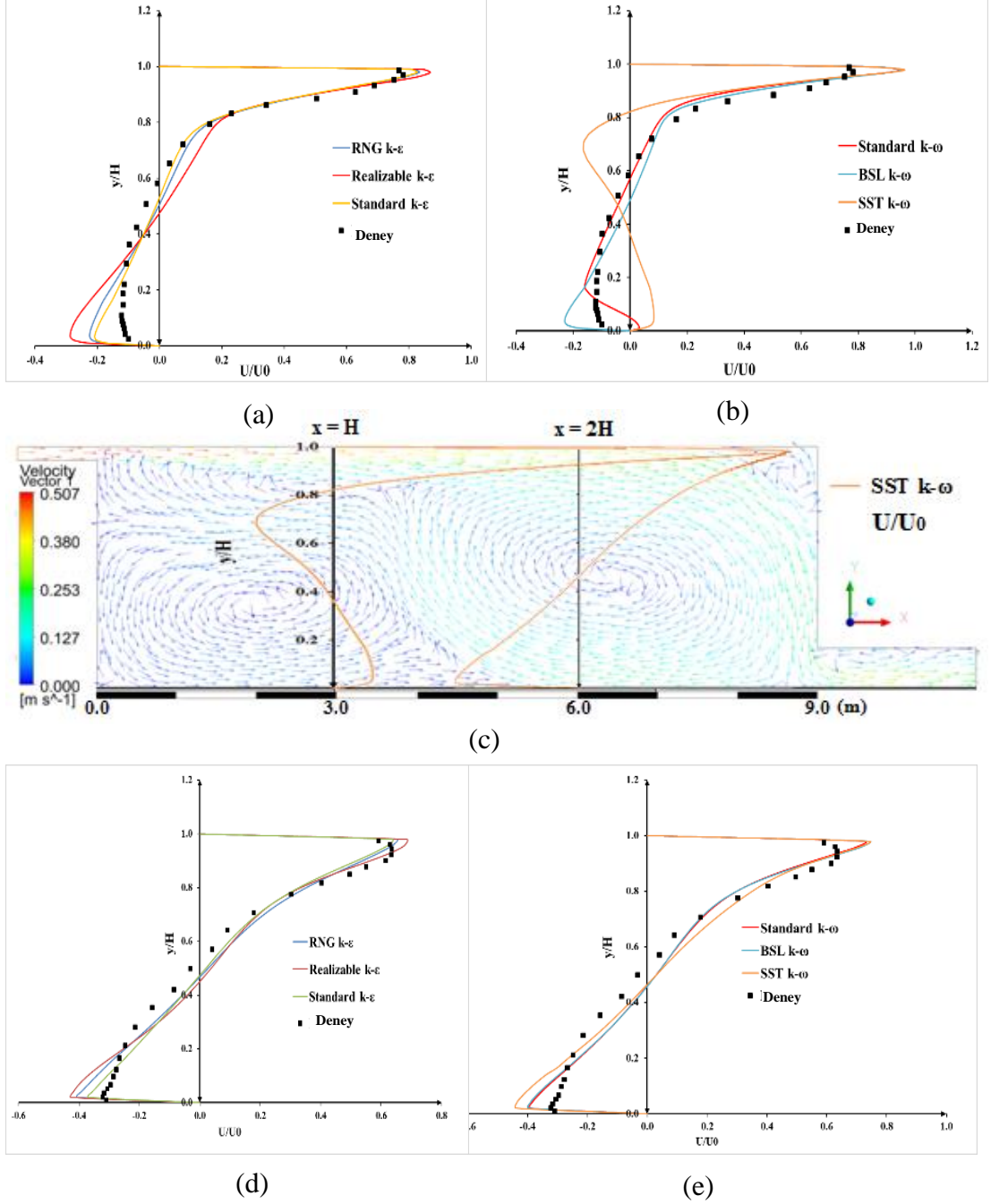
Şekil 4.5 Boyutsuz hızın x=H 'da x bileşeni for a) k-\epsilon modelleri, b) k-\omega modelleri, c) Hız vektörleri ve x=H ve x=2H 'da SST k-\omega modeliyle elde edilmiş U/U_0 boyutsuz hız profili, x=2H 'da boyutsuz hız profilleri a) k-\epsilon modelleri and b) k-\omega modelleri
