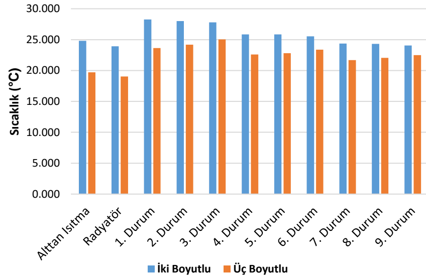
Şekil 4.25 Alttan ısıtma, radyatör ve klima ile ısıtmanın incelendiği iki boyutlu ve üç boyutlu çalışmalarda elde edilen ortalama oda sıcaklıkları.
