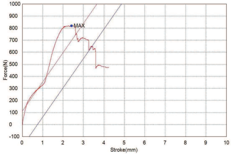
Şekil 4.19. Numune 8 Deney Kuvvet - Yer değiştirme
