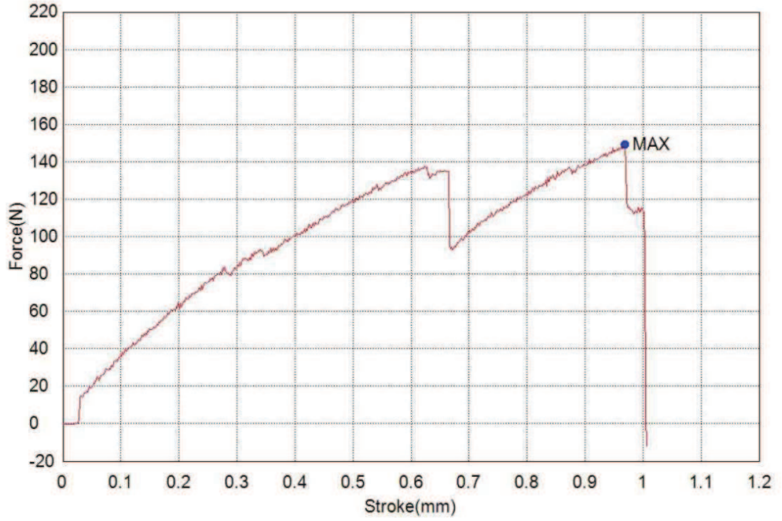
Şekil 4.6. Numune 1 Deney sonrasında elde edilen kuvvet yer değiştirme grafiği
