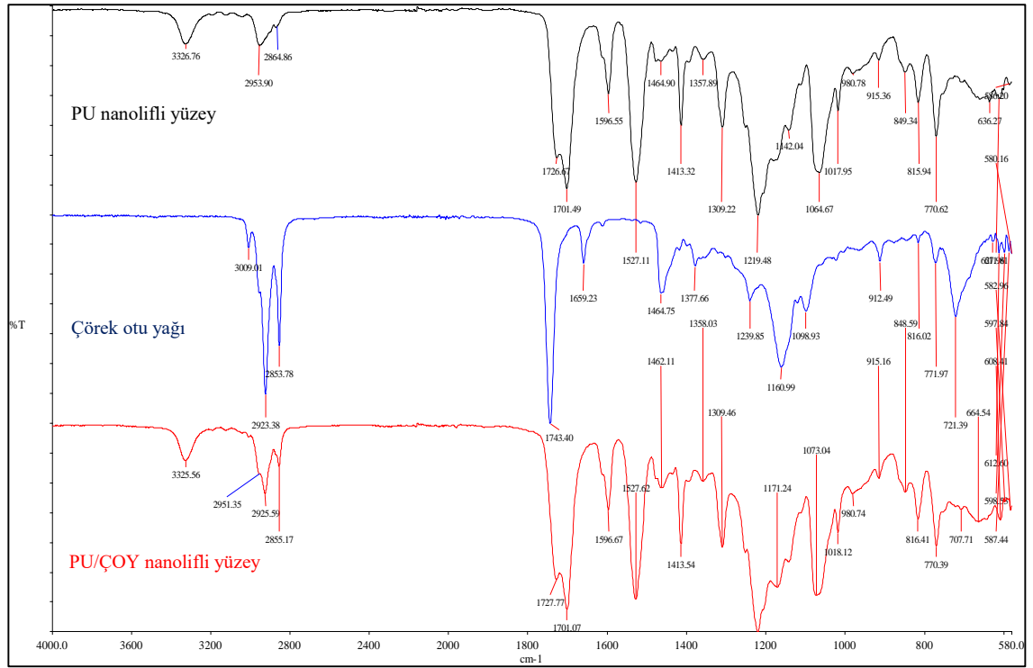
Şekil 4.4. ÇOY, PU nanolifli yüzey ve PU/ÇOY nanolifli yüzey FTIR spektrumu
