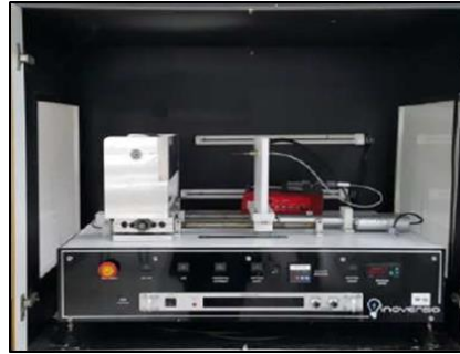
Şekil 3.9. Nanolifli yüzeylerin üretildiği elektro çekim ünitesi
