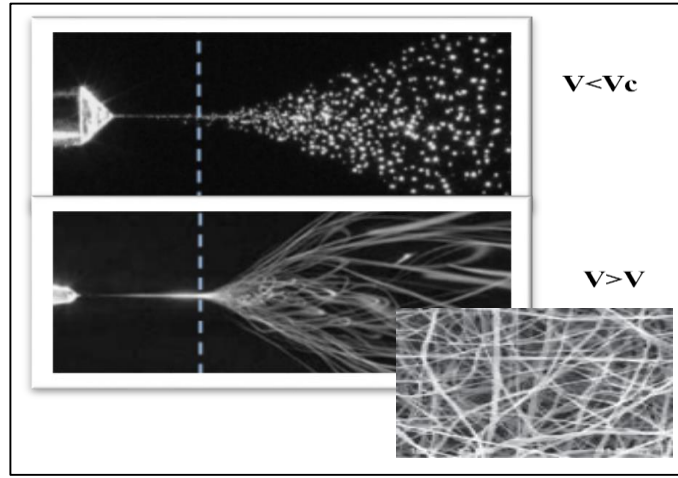
Şekil 2.15. Polimer jetinin whipping kararsızlığı davranışı ( https://www.nanoscience.com , 2019)
