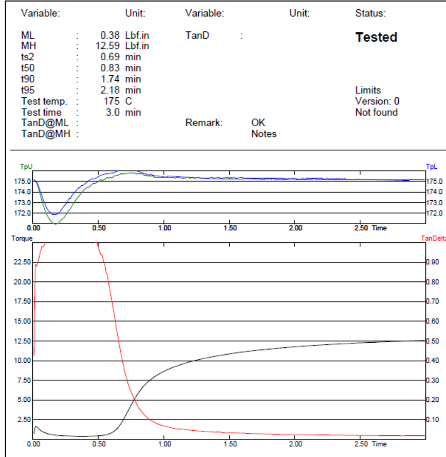
Şekil 3. 13. Kauçuk-Metal Yapıştırıcısının Rheometre Grafiği
