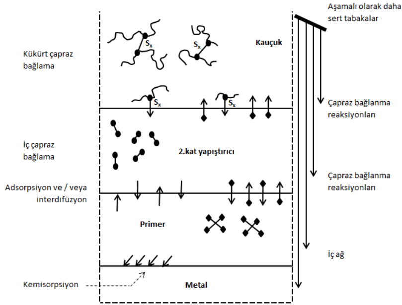
Şekil 2. 29. Vulkanizasyon bağlanma sürecinin şeması (Ebnesajjad 2008)
