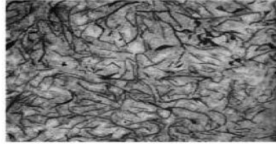
Şekil 2. 19. Lamel grafitli dökme demirler (Aran 2008)
