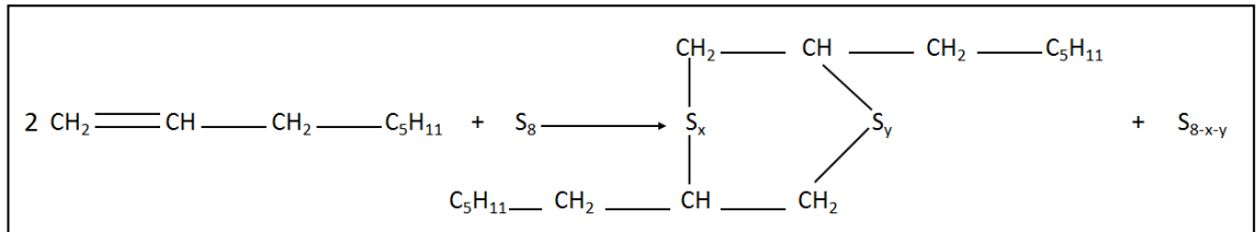
Şekil 2. 33. Çapraz bağlanma yapıları (Erkek 2007)
