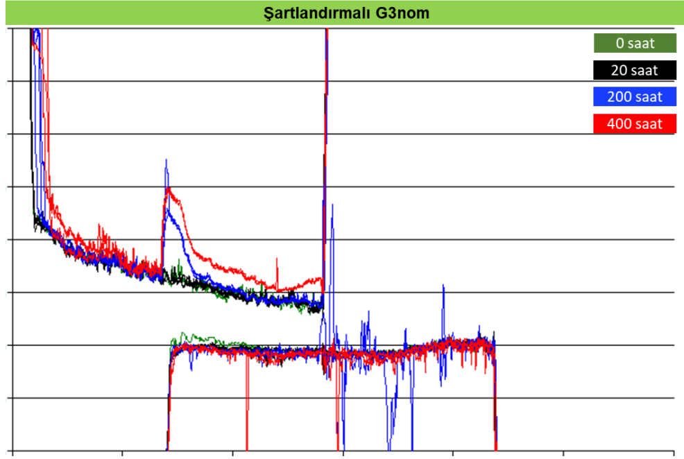
Şekil 4.8. 1. testte kullanılan şartlandırılmı G3nom varyantın iğne ve gövde oturma yüzeyi profilleri
