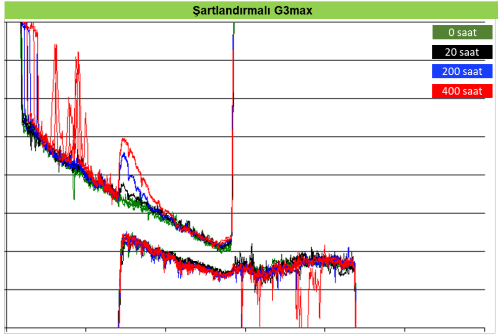
Şekil 4.15. 2. teste kullanılan şartlandırılmı G3max varyantın iğne ve gövde oturma yüzeyi profilleri
