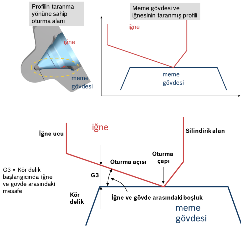
Şekil 2.16. Meme oturma yüzeyi profillerinin taranma oryantasyonu ve sonucunda oluşan görüntü (Bosch)
