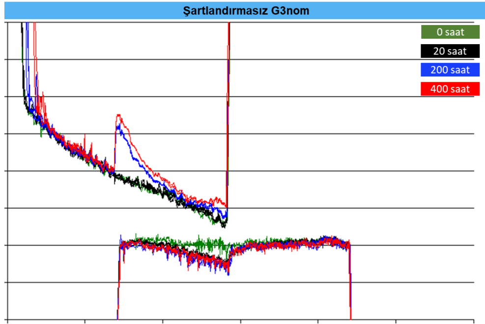
Şekil 4.5. 1. testte kullanılan şartlandırmasız G3nom varyantın iğne ve gövde oturma yüzeyi profilleri
