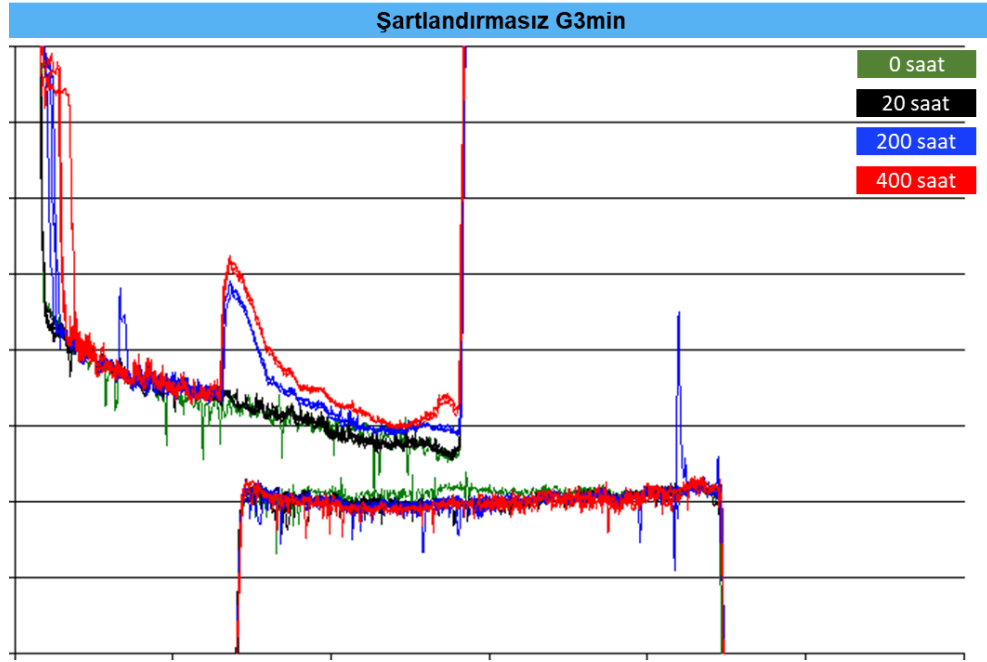
Şekil 4.4. 1. testte kullanılan şartlandırmasız G3min varyantın iğne ve gövde oturma yüzeyi profilleri
