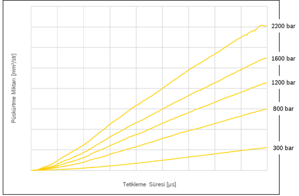
Şekil 3.22. Püskürtme karakteristiği eğrisi örneği
