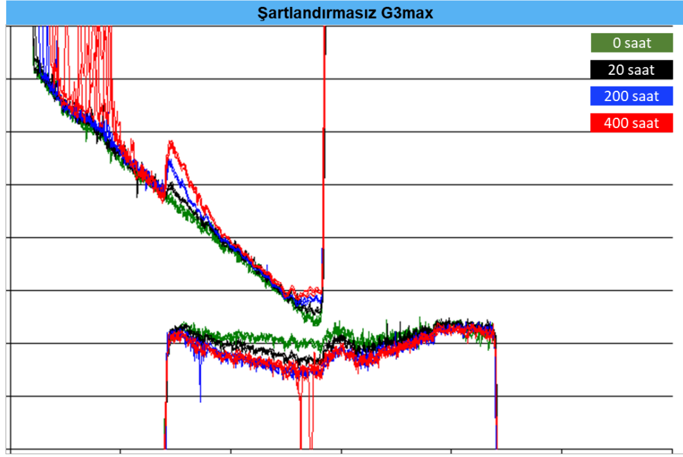
Şekil 4.12. 2. testte kullanılan şartlandırmasız G3max varyantın iğne ve gövde oturma yüzeyi profilleri
