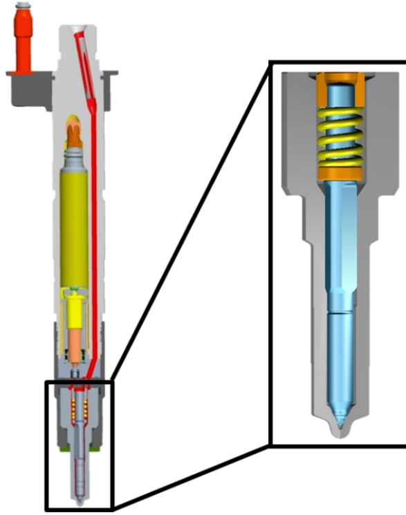
Şekil 2.12. Yeni tasarımın temelini oluşturan eski jenerasyonun 3 boyutlu modeli (Bosch)
