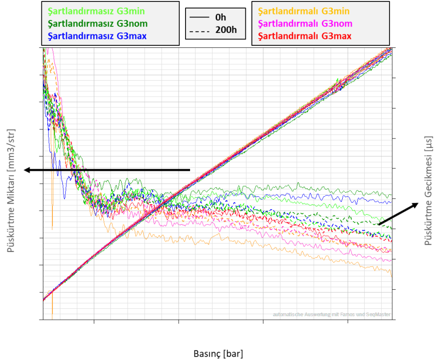
Şekil 4.26. 2. test 200 saat sonucunda püskürtme gecikmesi eğrisi
