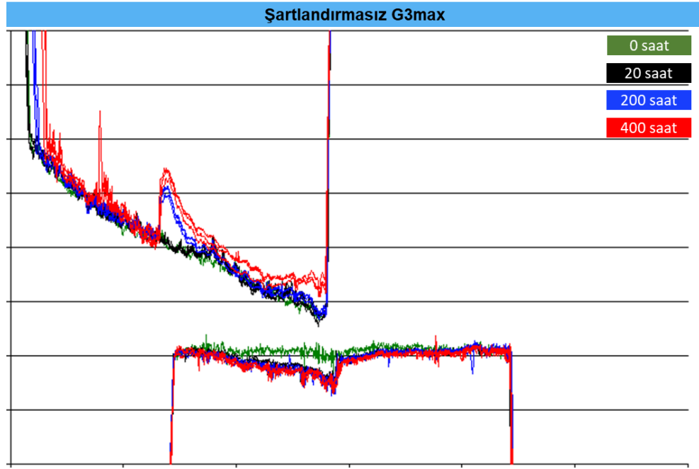
Şekil 4.6. 1. testte kullanılan şartlandırmasız G3max varyantın iğne ve gövde oturma yüzeyi profilleri
