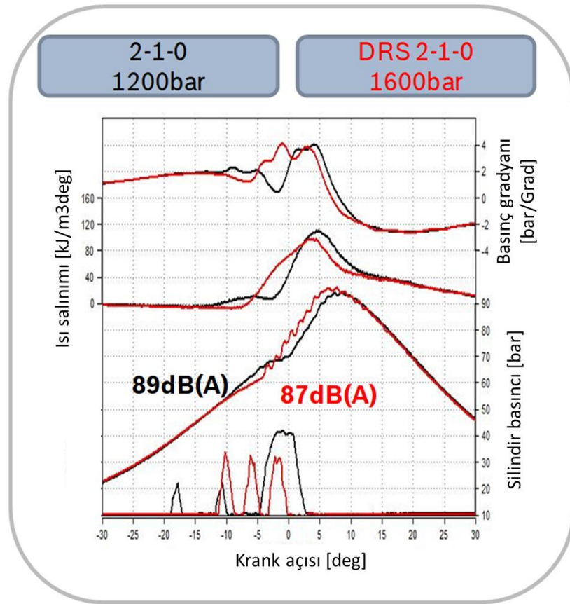
Şekil 2.10. Konvansiyonel ve DRS2 püskürtme düzenlerinin silindir basıncına ve ısı oluşumuna etkisi (Hammer ve ark. 2014)
