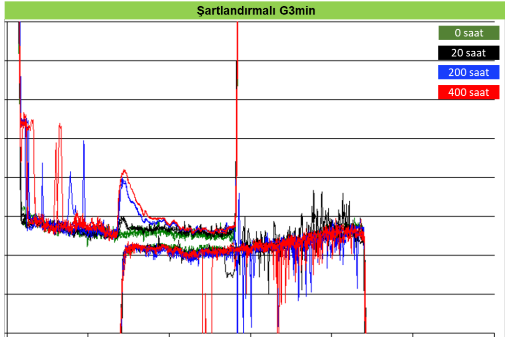
Şekil 4.13. 2. testte kullanılan şartlandırılmalı G3min varyantın iğne ve gövde oturma yüzeyi profilleri
