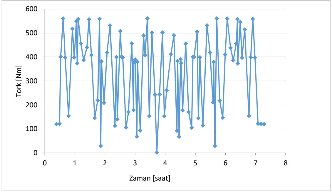
Şekil 3.8. Test sırasında ölçülen tork-zaman eğrisi
