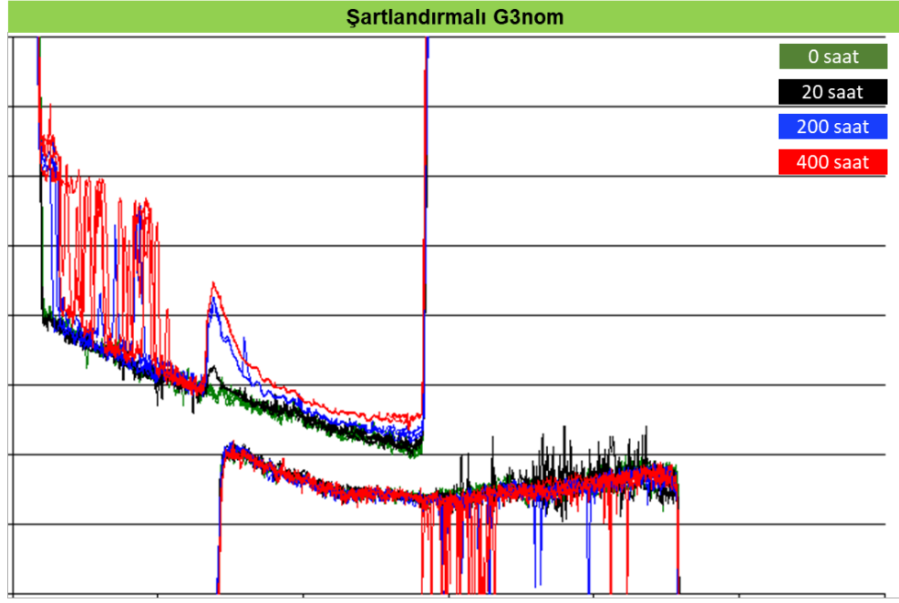
Şekil 4.14. 2. teste kullanılan şartlandırılmı G3nom varyantın iğne ve gövde oturma yüzeyi profilleri
