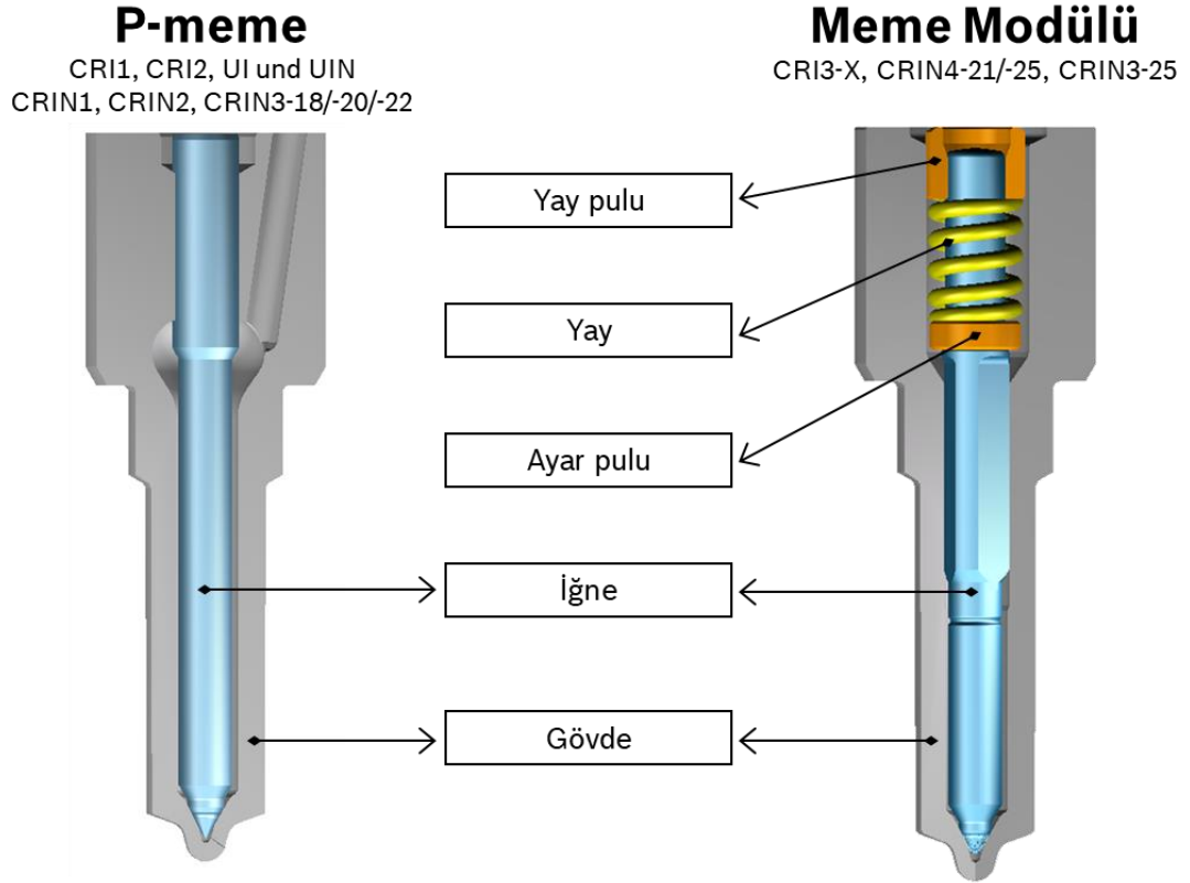
Şekil 2.7. Meme modülü ile P-meme arasındaki ana tasarım farkları (Bosch)
