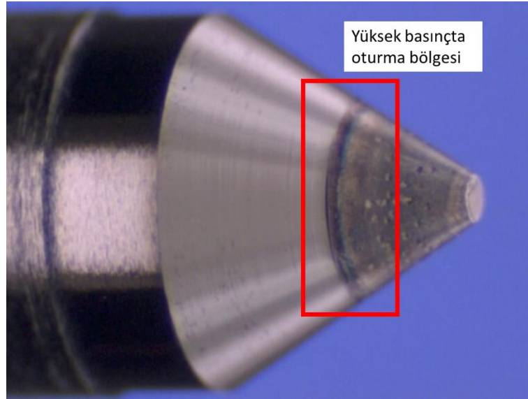
Şekil 4.1. İğne oturma yüzeyinde oluşan aşınma çizgisi
