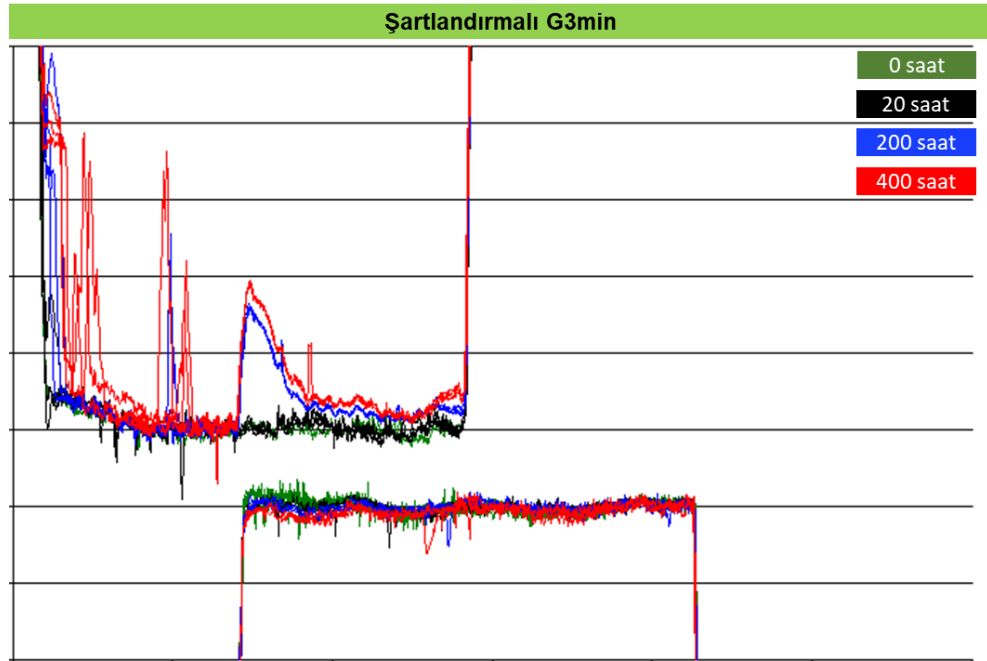
Şekil 4.7. 1. testte kullanılan şartlandırmalı G3min varyantın iğne ve gövde oturma yüzeyi profilleri
