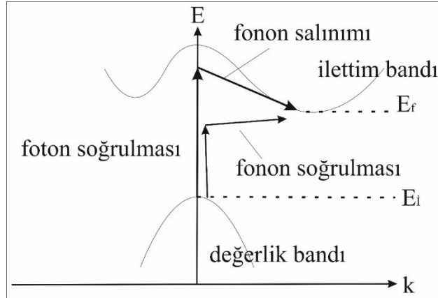
Şekil 2.8. Yarıiletken bir malzemenin dolaylı bant geçişi.
