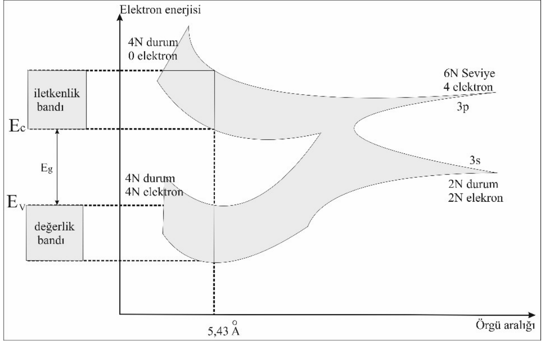
Şekil 2.11. N tane oturun bir araya gelerek Si kristalinin oluşturulmasının şematik gösterimi.
