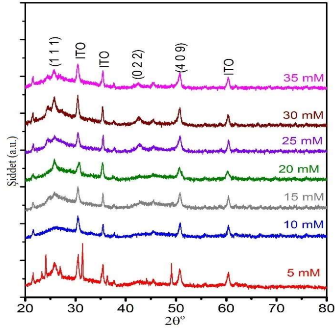
Şekil 4. 9. ITO alttaşlar üzerine büyütülmüş In:CdSe ince filmlerin XRD grafikleri.
