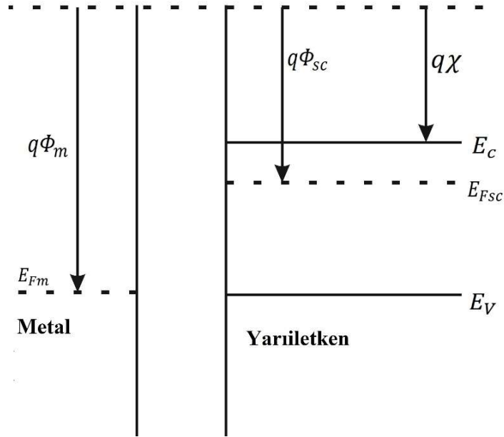
Şekil 2.15. Bir metal ve yarıiletkene ait bant yapılarının şematik gösterimi.
