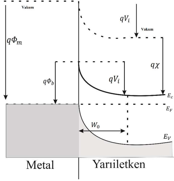
Şekil 2.16. Bir Schottky diyotun enerji bant diyagramının şematik gösterimi.
