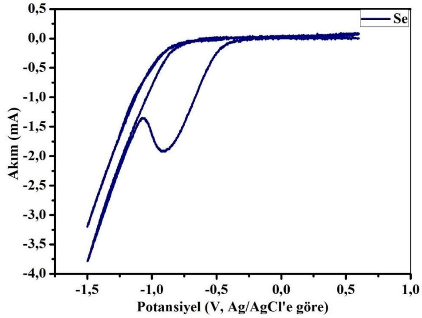
Şekil 3.13. Se elementine ait çözeltinin döngüsel voltammogram grafiği.
