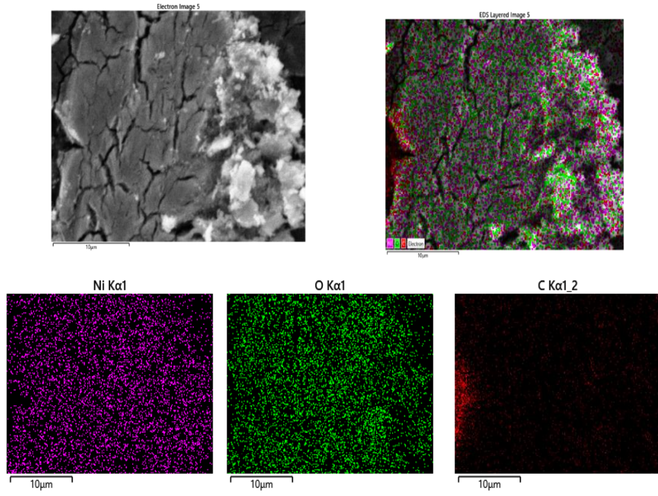
Şekil 4.25. pH = 4,1 değerine sahip filmin yüzey haritalama görüntüleri
