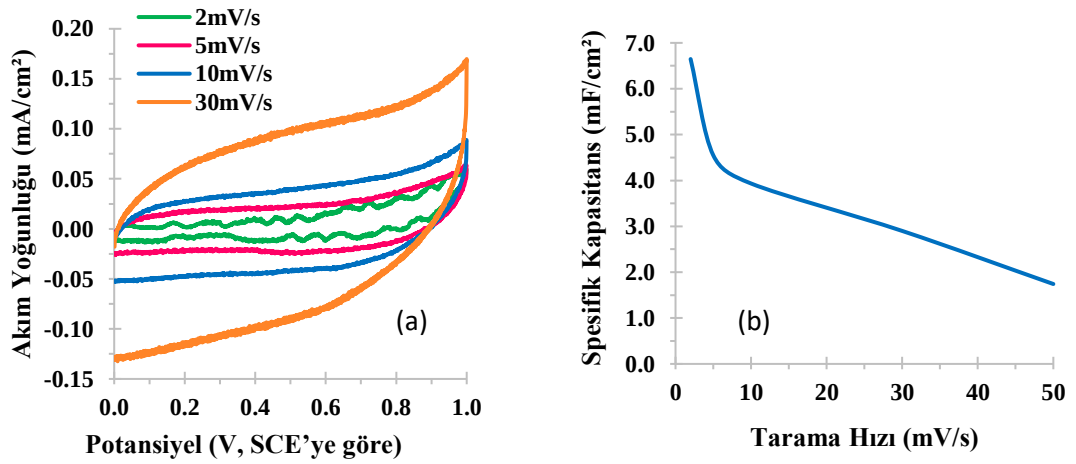
Şekil 4.17. (a) pH = 4,1 değerine sahip filmin \text{Na}_2\text{SO}_4 çözeltisinde kapasitans grafiği (b) pH = 4,1 değerine sahip filmin \text{Na}_2\text{SO}_4 çözeltisindeki kapasitif davranışından edilen grafikten hesaplanan spesifik kapasitans değerleri
