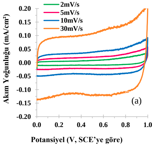
Şekil 4.21. (a) pH = 6,3 değerine sahip filmin \text{Na}_2\text{SO}_4 çözeltisinde kapasitans grafiği (b) pH = 6,3 değerine sahip filmin \text{Na}_2\text{SO}_4 çözeltisindeki kapasitif davranışından edilen grafikten hesaplanan spesifik kapasitans değerleri
