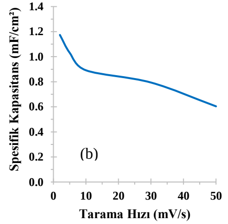
Şekil 4.20. (a) pH = 5,6 değerine sahip filmin \text{Na}_2\text{SO}_4 çözeltisinde kapasitans grafiği (b) pH = 5,6 değerine sahip filmin \text{Na}_2\text{SO}_4 çözeltisindeki kapasitif davranışından edilen grafikten hesaplanan spesifik kapasitans değerleri
