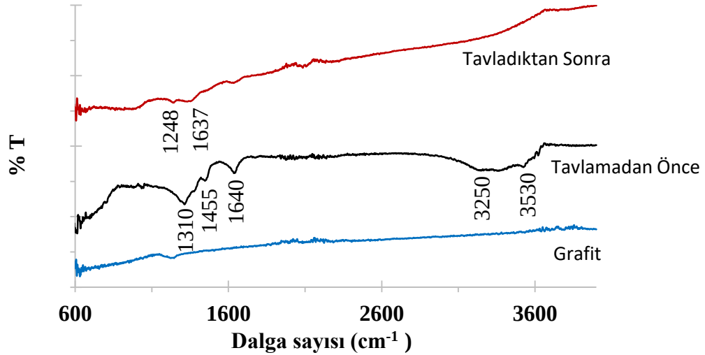
Şekil 4.4. Grafit Alttabakanın, Nikel-hidroksit ve Ni-oksit filmlerin FTIR spektrumu
