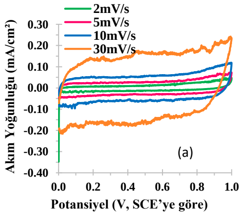
Şekil 4.19. (a) pH = 5,1 değerine sahip filmin \text{Na}_2\text{SO}_4 çözeltisinde kapasitans grafiği (b) pH = 5,1 değerine sahip filmin \text{Na}_2\text{SO}_4 çözeltisindeki kapasitif davranışından edilen grafikten hesaplanan spesifik kapasitans değerleri
