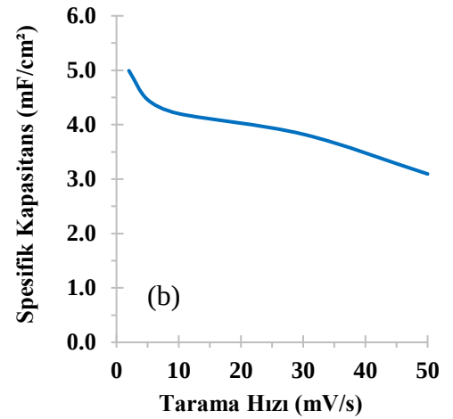
Şekil 4.21. (a) pH = 6,3 değerine sahip filmin \text{Na}_2\text{SO}_4 çözeltisinde kapasitans grafiği (b) pH = 6,3 değerine sahip filmin \text{Na}_2\text{SO}_4 çözeltisindeki kapasitif davranışından edilen grafikten hesaplanan spesifik kapasitans değerleri
