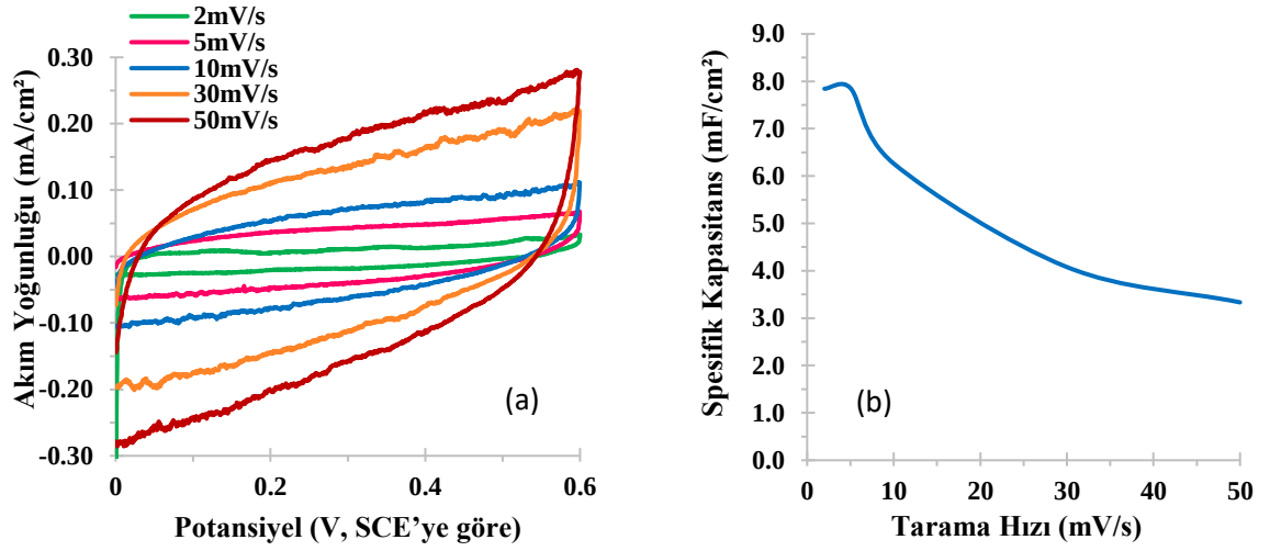
Şekil 4.13. (a) pH = 4,1 değerine sahip filmin \text{Na}_2\text{SO}_4 çözeltisinde kapasitif davranışı (b) pH = 4,1 değerine sahip filmin \text{Na}_2\text{SO}_4 çözeltisindeki kapasitif davranışından elde edilen grafikten hesaplanan spesifik kapasitans değerleri
