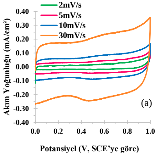
Şekil 4.18. (a) pH = 4,6 değerine sahip filmin \text{Na}_2\text{SO}_4 çözeltisinde kapasitans grafiği (b) pH = 4,6 değerine sahip filmin \text{Na}_2\text{SO}_4 çözeltisindeki kapasitif davranışından edilen grafikten hesaplanan spesifik kapasitans değerleri
