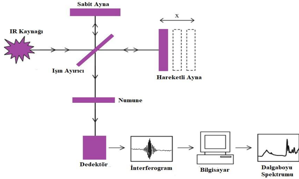
Şekil 3.7. FTIR şematik görüntüsü
