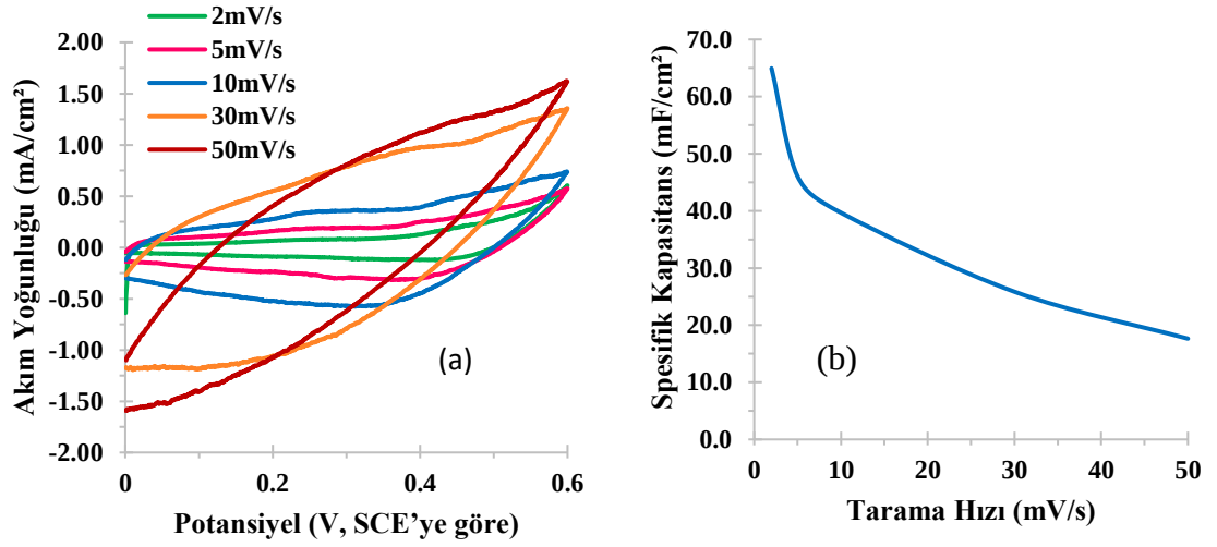
Şekil 4.10. (a) 300 °C' de 2 saat tavlanan filme ait akım yoğunluğu-potansiyel grafiği (b) Akım yoğunluğu potansiyel grafiğinden elde edilerek hesaplanan spesifik kapasitans değeri
