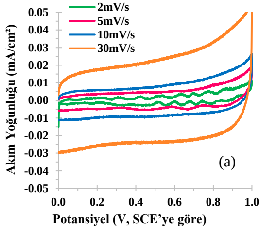
Şekil 4.20. (a) pH = 5,6 değerine sahip filmin \text{Na}_2\text{SO}_4 çözeltisinde kapasitans grafiği (b) pH = 5,6 değerine sahip filmin \text{Na}_2\text{SO}_4 çözeltisindeki kapasitif davranışından edilen grafikten hesaplanan spesifik kapasitans değerleri
