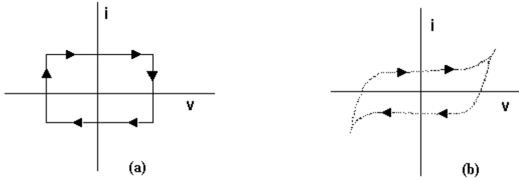
Şekil 3.5. (a) İdeal bir kondansatörün CV eğrisi (b) Gerek bir kondansatörün CV eğrisi
