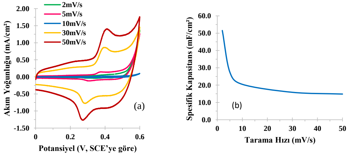
Şekil 4.9. (a) 300 °C' de 1 saat tavlanan filme ait akım yoğunluğu-potansiyel grafiği (b) Akım yoğunluğu potansiyel grafiğinden elde edilerek hesaplanan spesifik kapasitans değeri
