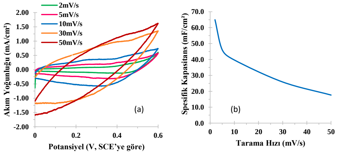
Şekil 4.12. (a) pH = 4,1 değerine sahip filmin KOH çözeltisinde kapasitif davranışı (b) pH = 4,1 değerine sahip filmin KOH çözeltisindeki kapasitif davranışından edilen grafikten hesaplanan spesifik kapasitans değerleri
