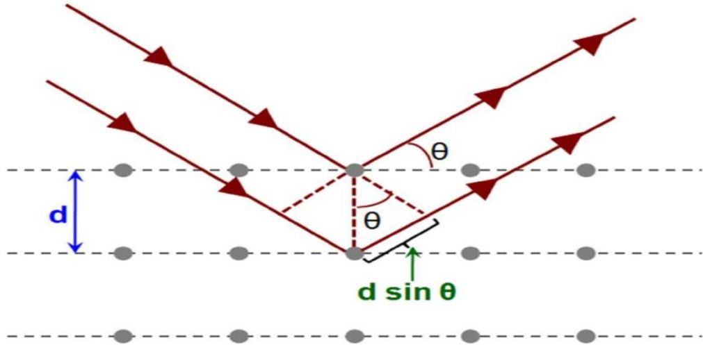
Şekil 3.9. Bragg kırınımı
