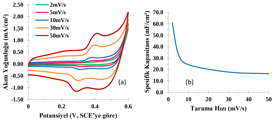
Şekil 4.11. (a) 300 °C' de 3 saat tavlanan filme ait akım yoğunluğu-potansiyel grafiği (b) Akım yoğunluğu potansiyel grafiğinden elde edilerek hesaplanan spesifik kapasitans değeri
