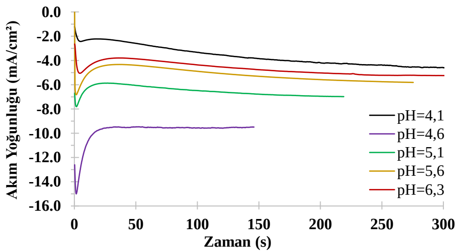
Şekil 4.3. Farklı pH değerlerinde \text{Ni}(\text{OH})_2 film üretimi sırasında kaydedilen akım yoğunluğu-zaman grafikleri
