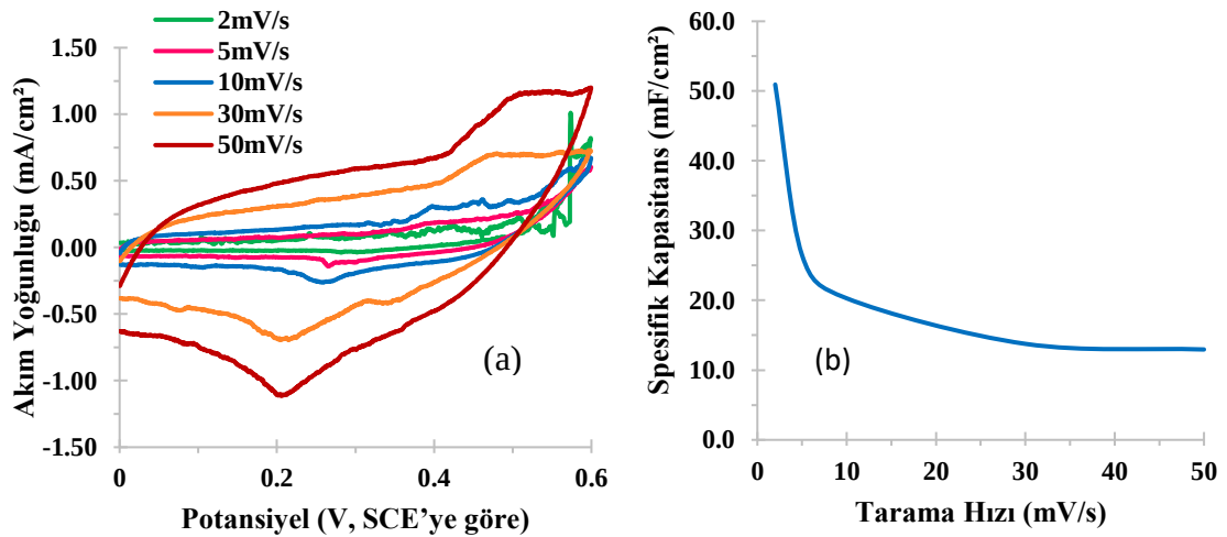
Şekil 4.15. (a) pH = 6,3 değerine sahip filmin KOH çözeltisinde kapasitif davranışı (b) pH = 6,3 değerine sahip filmin KOH çözeltisindeki kapasitif davranışından edilen grafikten hesaplanan spesifik kapasitans değerleri
