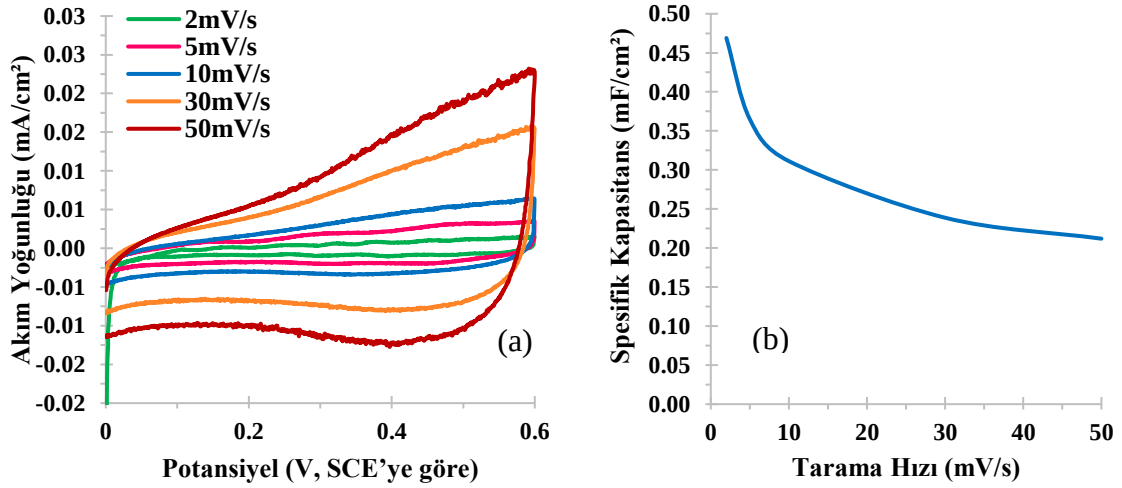
Şekil 4.14. (a) pH = 4,1 değerine sahip filmin \text{H}_2\text{SO}_4 çözeltisinde kapasitif davranışı (b) pH = 4,1 değerine sahip filmin \text{H}_2\text{SO}_4 çözeltisindeki kapasitif davranışından elde edilen grafikten hesaplanan spesifik kapasitans değerleri
