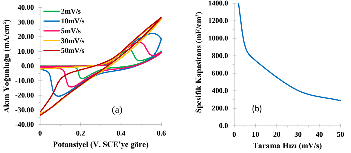
Şekil 4.8. (a) Tavlanmayan filme ait akım yoğunluğu-potansiyel grafiği (b) Akım yoğunluğu-potansiyel grafiğinden elde edilerek hesaplanan spesifik kapasitans grafikleri
