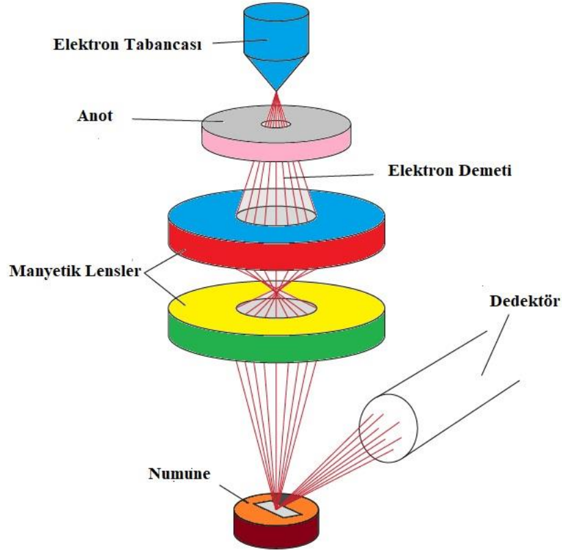
Şekil 3.10. SEM'in şematik görüntüsü
