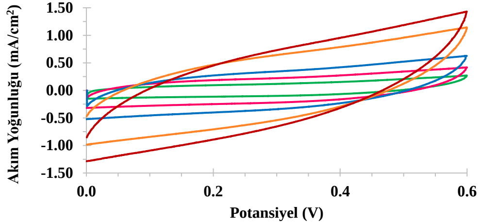
Şekil 4.7. Grafıt alttabaka için kapasitans grafiđi
