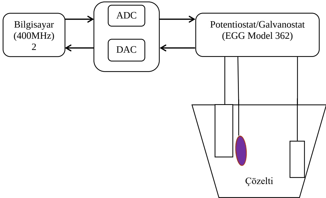
Şekil 3.4. Elektrodepozisyon yöntemi için kullanılan düzeneğin şeması
