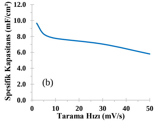
Şekil 4.18. (a) pH = 4,6 değerine sahip filmin \text{Na}_2\text{SO}_4 çözeltisinde kapasitans grafiği (b) pH = 4,6 değerine sahip filmin \text{Na}_2\text{SO}_4 çözeltisindeki kapasitif davranışından edilen grafikten hesaplanan spesifik kapasitans değerleri
