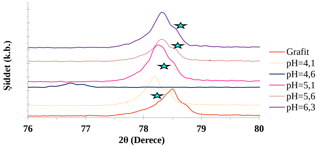
Şekil 4.6. 78,5 °C’de farklı pH değerleri için XRD desenleri
