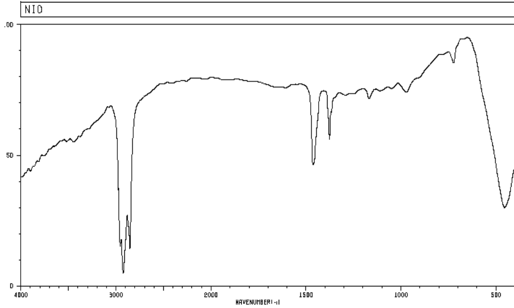
Şekil 3.8. NiO için FTIR spektroskopisi ( https://sdb.sdb.aist.go.jp/sdb/cgi-bin/cre_index.cgi )
