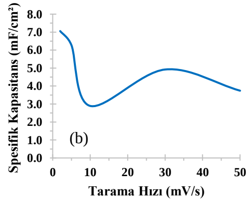
Şekil 4.19. (a) pH = 5,1 değerine sahip filmin \text{Na}_2\text{SO}_4 çözeltisinde kapasitans grafiği (b) pH = 5,1 değerine sahip filmin \text{Na}_2\text{SO}_4 çözeltisindeki kapasitif davranışından edilen grafikten hesaplanan spesifik kapasitans değerleri
