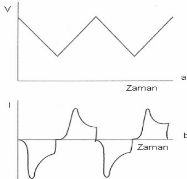
Şekil 3.2. (a) Dönüşümlü voltamogramın elde edilmesinde kullanılan potansiyelin zamanla değişimi (b) Bu potansiyele karşılık gelen akım değişimi (Hibbert 1993)
