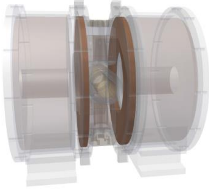
Şekil 2.26. Sürücü alanı z yönündeki jeneratörünün bobin montajı (Viereck 2016).
