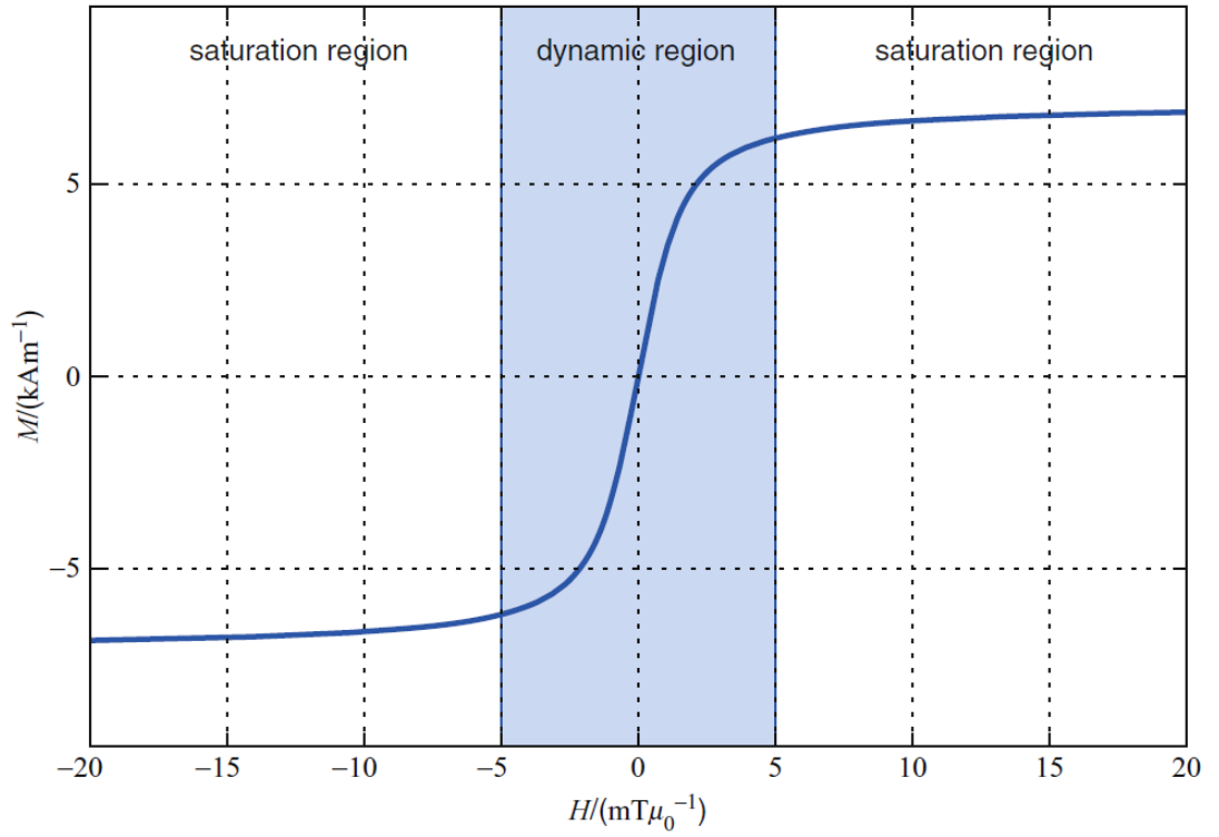
Şekil 2.4. Dış manyetik alan küçük ise, parçacıklar doyumda değildir ve mıknatıslanma keskin bir artış gösterir. Daha büyük dış alanlar için, parçacık doyuma girer ve mıknatıslanma dış alanla daha zor değişir (Knopp ve Buzug 2012).
