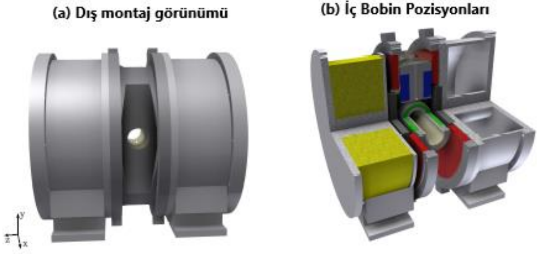
Şekil 2.22. Sürücü alanı bobinleri, x (yeşil), y (mavi) ve z ekseni (kırmızı) için alan jeneratörlerini göstermek üzere renklendirilir. Gradyan bobinleri, siyah renkte sabit mıknatıslarla sarı renkte gösterilmiştir (Viereck 2016).
