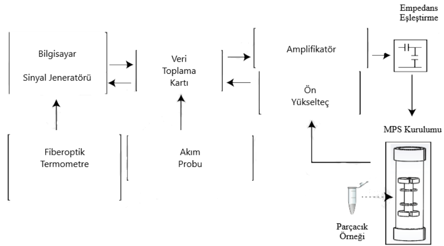
Şekil 2.13. Genel MPS deney akış göstergesi.
