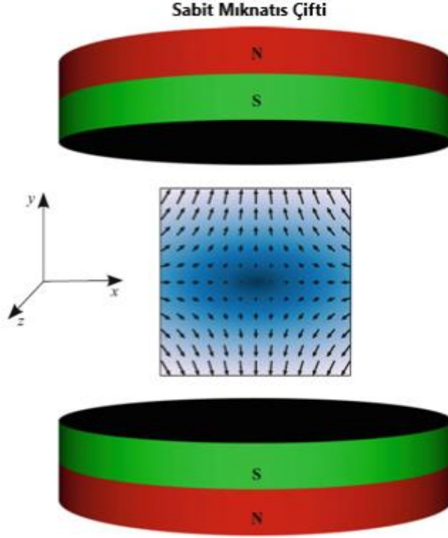
Şekil 2.20. Bir MAN gradyan alanının kurulacağı şekilde güney direkleri ile birbirine bakan iki sabit mıknatıs. Kuzey kutbu kırmızı renkte iken güney kutbu yeşil renktedir (Knopp ve Buzug 2012).
