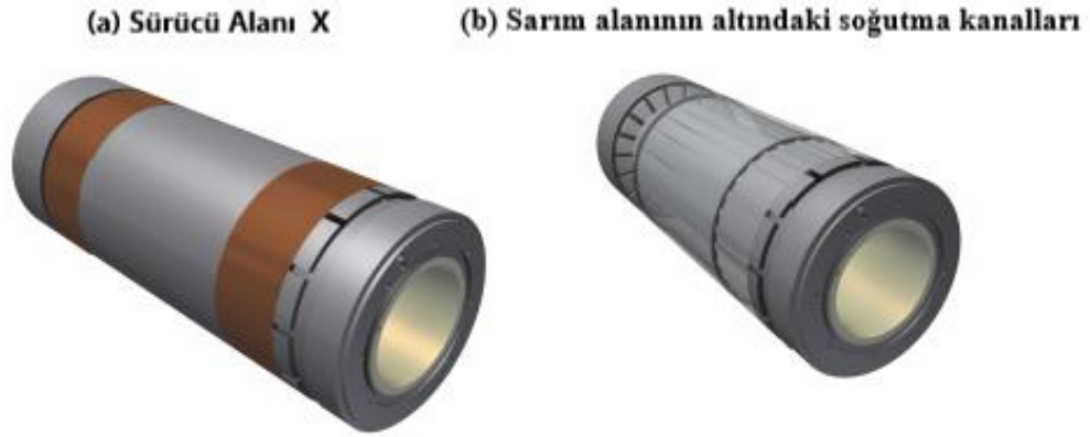
Şekil 2.24. X sürücü alan jeneratörünün ve gömülü soğutma kanalları (Viereck 2016).
