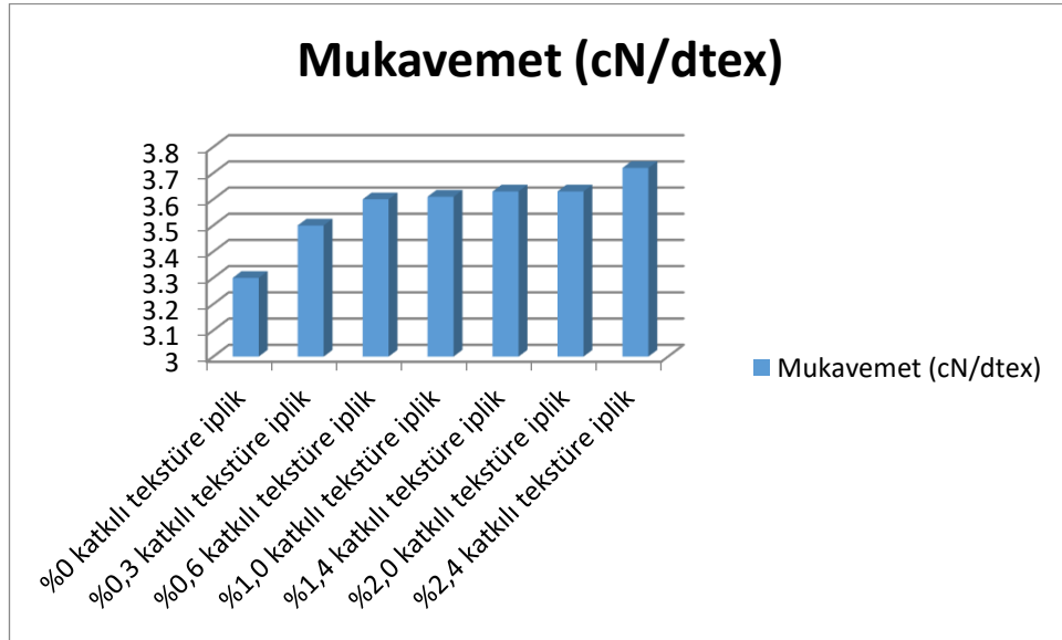
Şekil 5.7. Tekstüre ipliklerin mukavemet (cN/dtex) sonuçları
