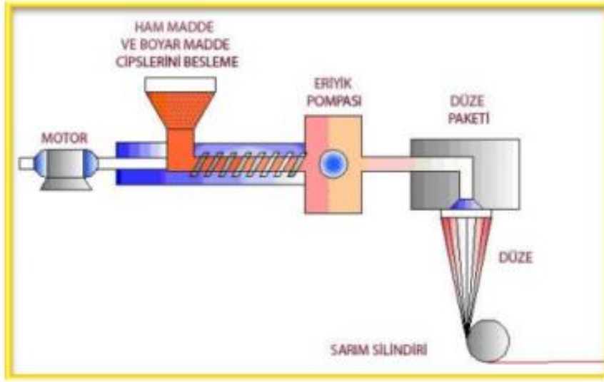
Şekil 2.7. Eriyikten lif üretiminde katkı maddesi eklenmesi (Kozanoğlu 2006)
