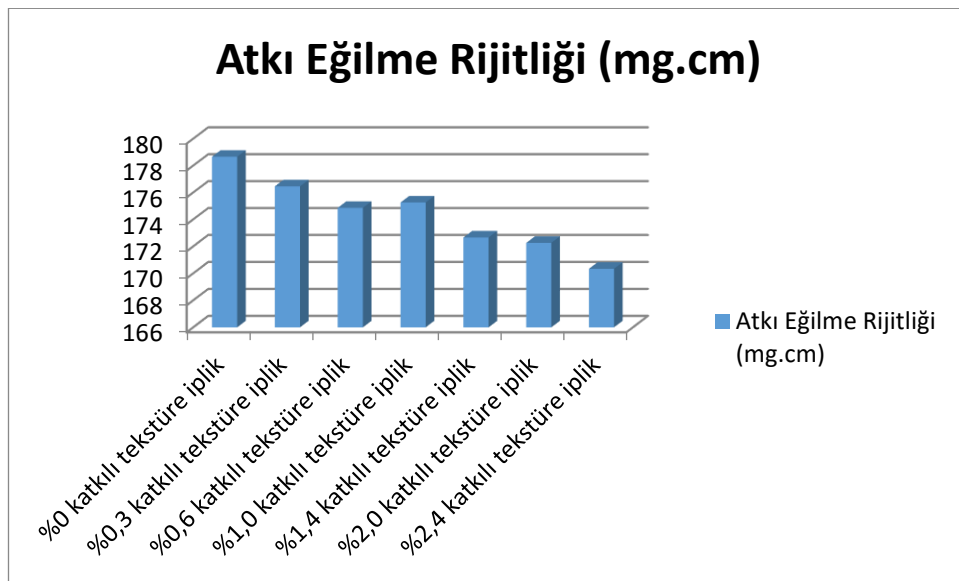
Şekil 5.18. Dokuma kumaşların atkı eğilme rijitliği (mg.cm) sonuçları
