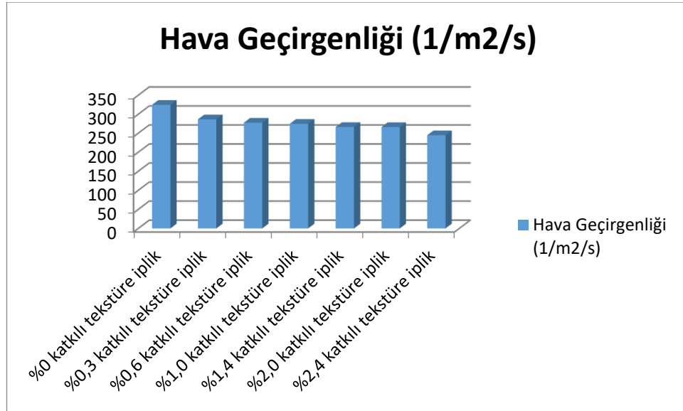
Şekil 5.13. Dokuma kumaşların hava geçirgenliği (1/m 2 /s) sonuçları
