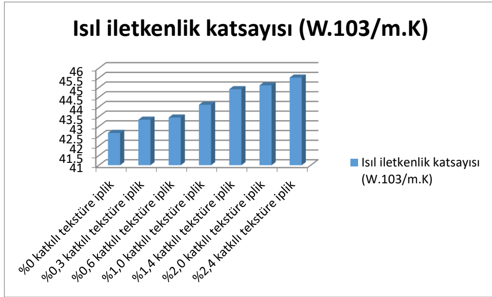
Şekil 5.14. Dokuma kumaşların ısı iletkenlik katsayısı (W.10 3 /m.K) sonuları
