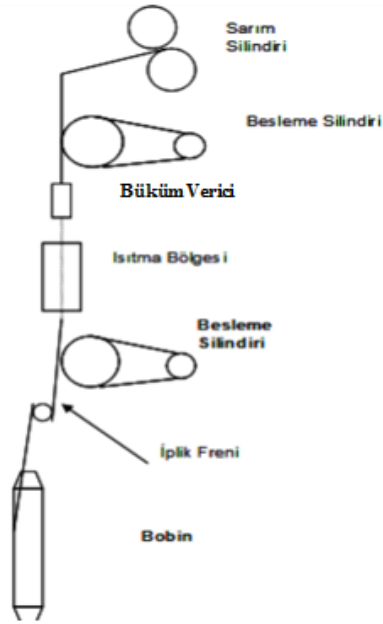
Şekil 2.8. Yalancı büküm tekstüre işlemi (Çirkin 2006)
