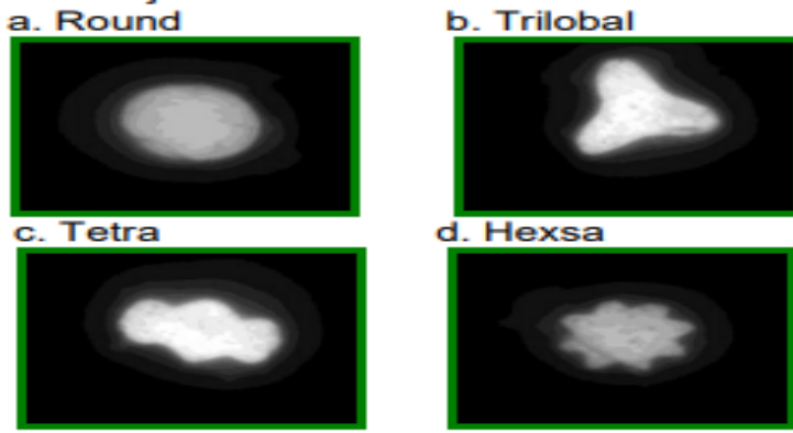
Şekil 2.6. Farklı kesitlerdeki filamentlerin lif enine kesit görüntüleri (Özkan 2008)
