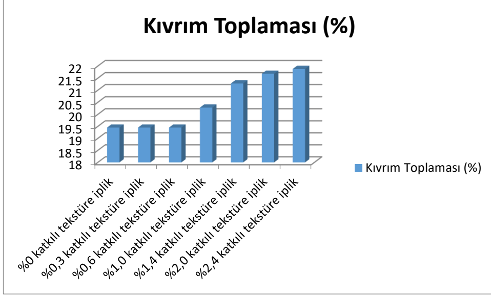
Şekil 5.4. Tekstüre ipliklerin kıvrım toplamaları (%) sonuçları
