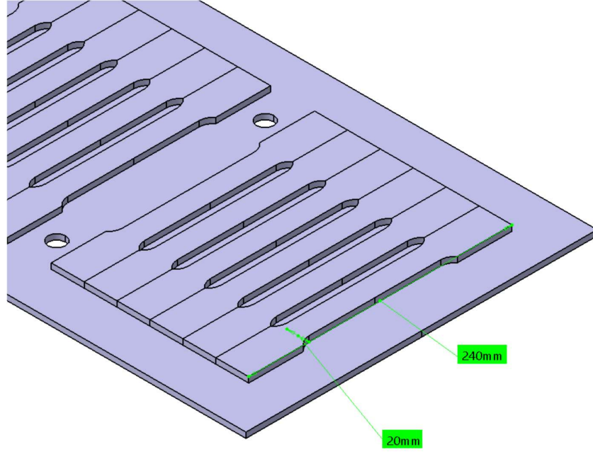
Şekil 3.13. Metalik Malzemelerin Çekme Deney Standardı EN ISO 6892' ye uygun çekme numuneleri şematik gösterimi.
