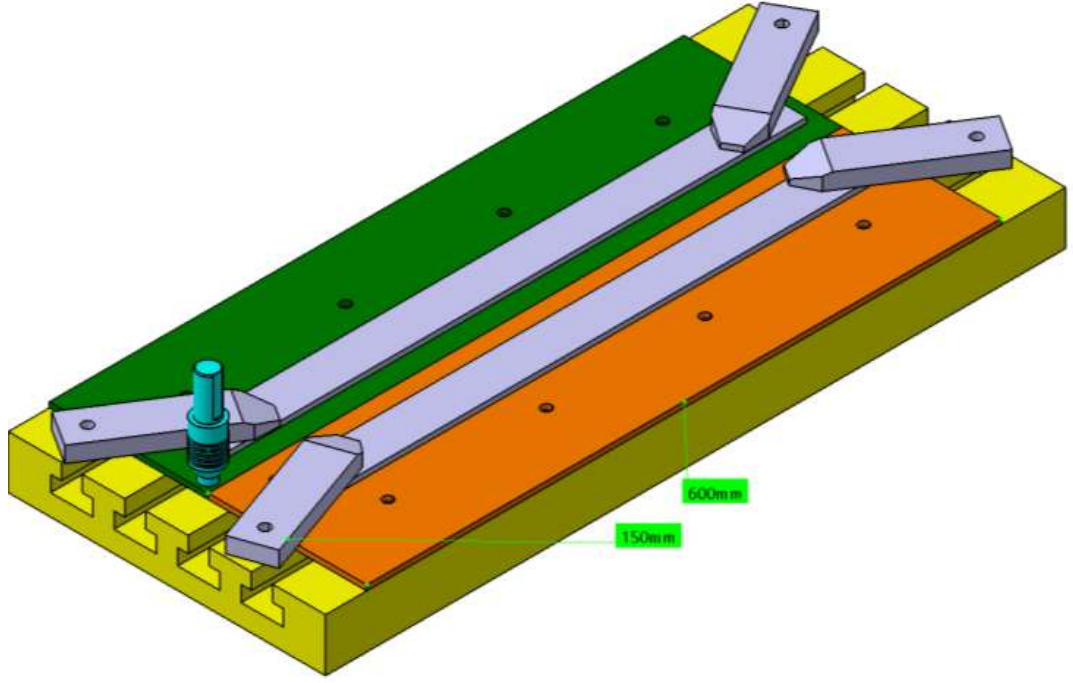
Şekil 3.1. Kullanılan plakaların şematik gösterimi.
