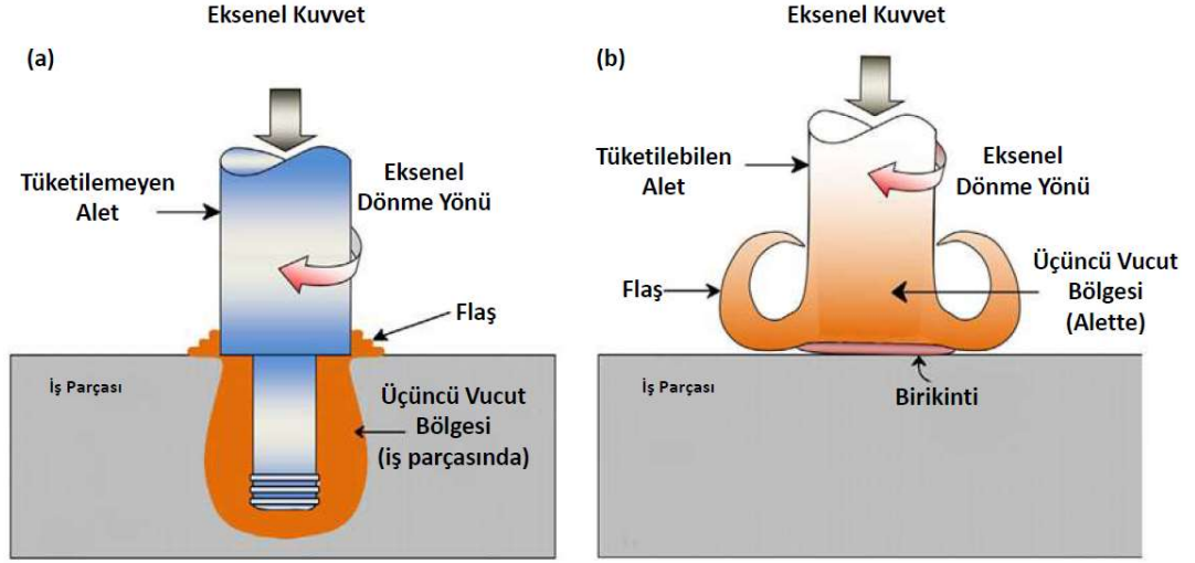
Şekil 1.2. Sürtünme karıştırma işlemlerinde üçüncü vücut bölgesi ile (a) Sürtünme karıştırma kaynağında olduğu gibi sarf malzeme olmayan uç (b) Sürtünme yüzeyinde olduğu gibi sarf malzeme olan uç (G.K. Padhy, C.S. Wu*, S. Gao 2018).
