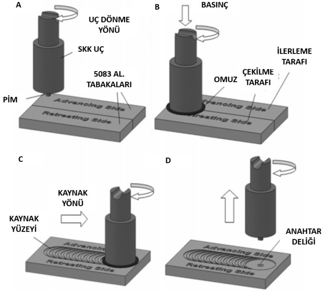
Şekil 2.3. FSW işleminin dört aşamasının şematik gösterimi: (A) Dalma Aşaması, (B) Bekleme Aşaması, (C) Kaynak ve (D) Geri Çekme/Soğutma Aşaması (AO Mosleh ve ark. 2015).
