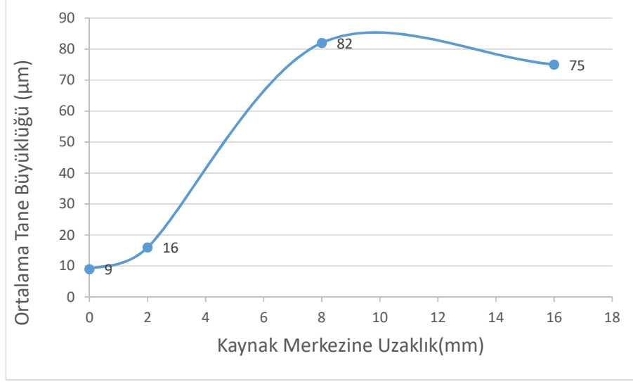
Şekil 4.21. 8. kaynağın merkezden itibaren ortalama tane büyüklükleri (µm).
