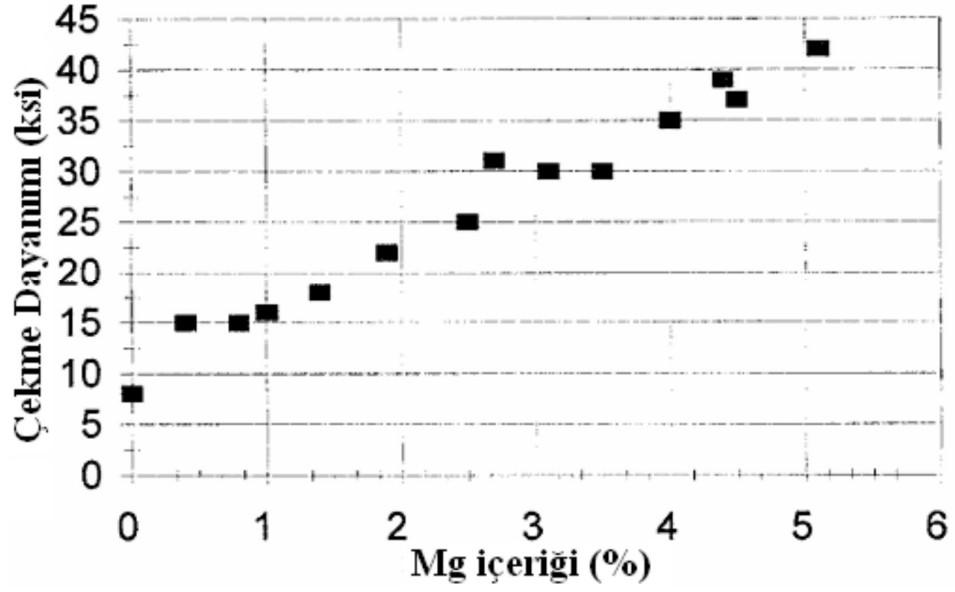
Şekil 2.5. Artan Mg içeriği ile değişen gerilme dayanımı (Kissel ve Ferry 2002).
