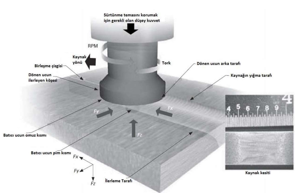
Şekil 2.1. Sürtünme karıştırma işleminin şematik gösterimi (H. Tarık Serindağ 2014) .
