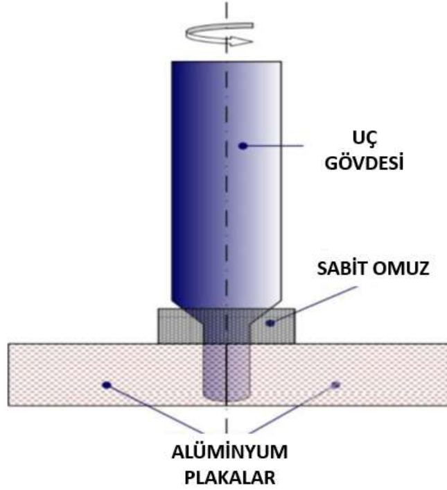
Şekil 2.6. Sabit omuzlu sürtünme karıştırma kaynağının şematik gösterimi (J. Martin 2017).
