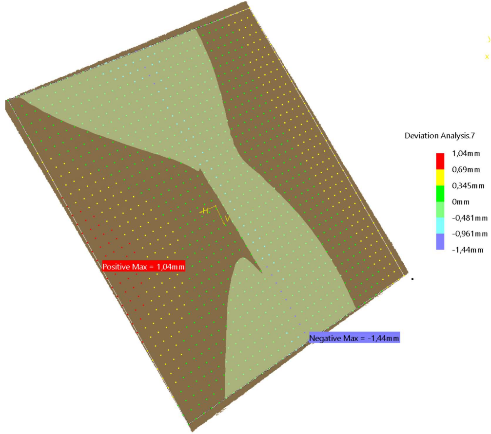
Şekil 4.33. TIG kaynağı yüzey taraması sonucu.
