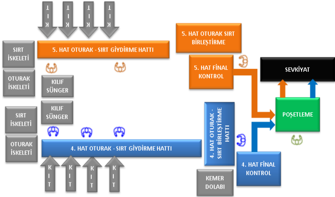
Şekil 4.9. İyileştirme sonrası yerleşim düzeni
