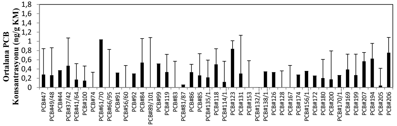
Şekil 4.10. GA Örnekleme Noktasında PCB Tür Dağılımı
