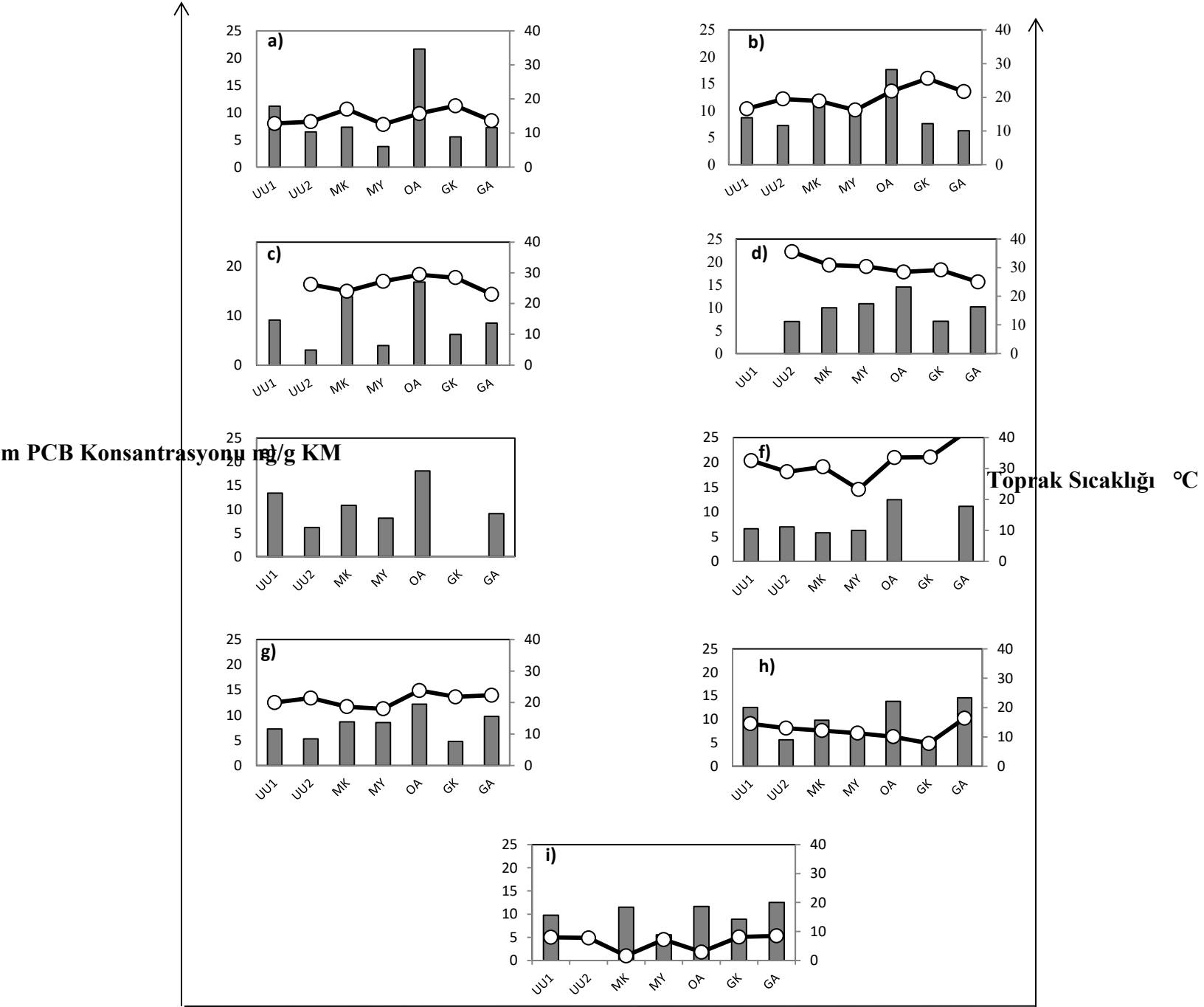
Şekil 4.2. Örneklem noktalarına göre PCB Konsantrasyonları ve Sıcaklık Değerleri
