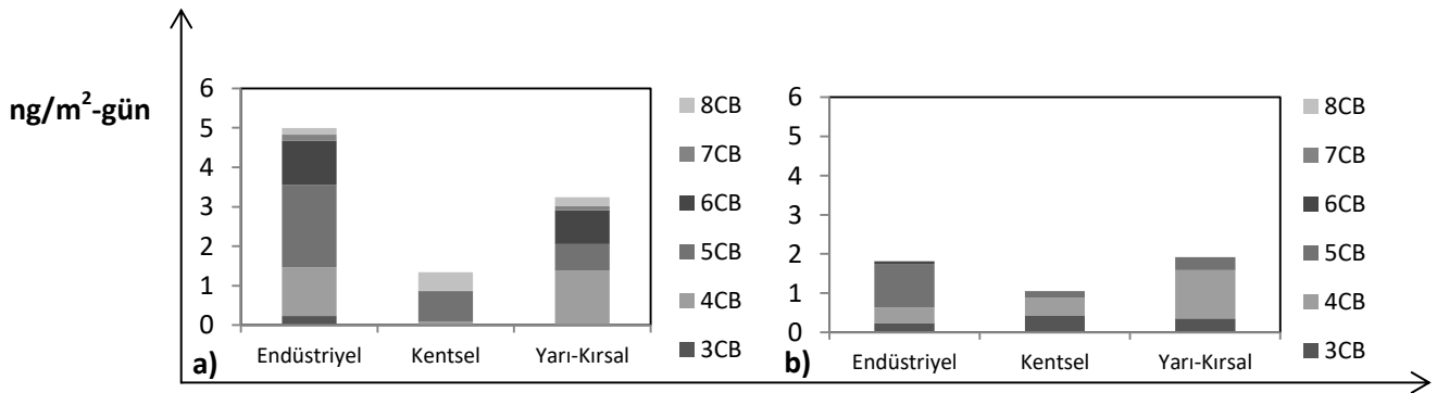
Şekil 4.20. Bölgesel Net Akı Değerlerinde PCB Homolog Dağılımları a) Yaz b) Kış
