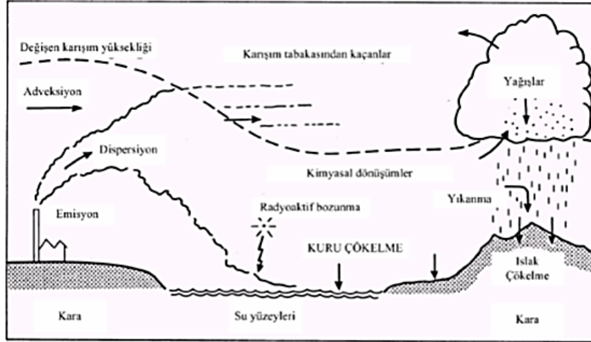
Şekil 2.2. Atmosferik çökeltme süreci
