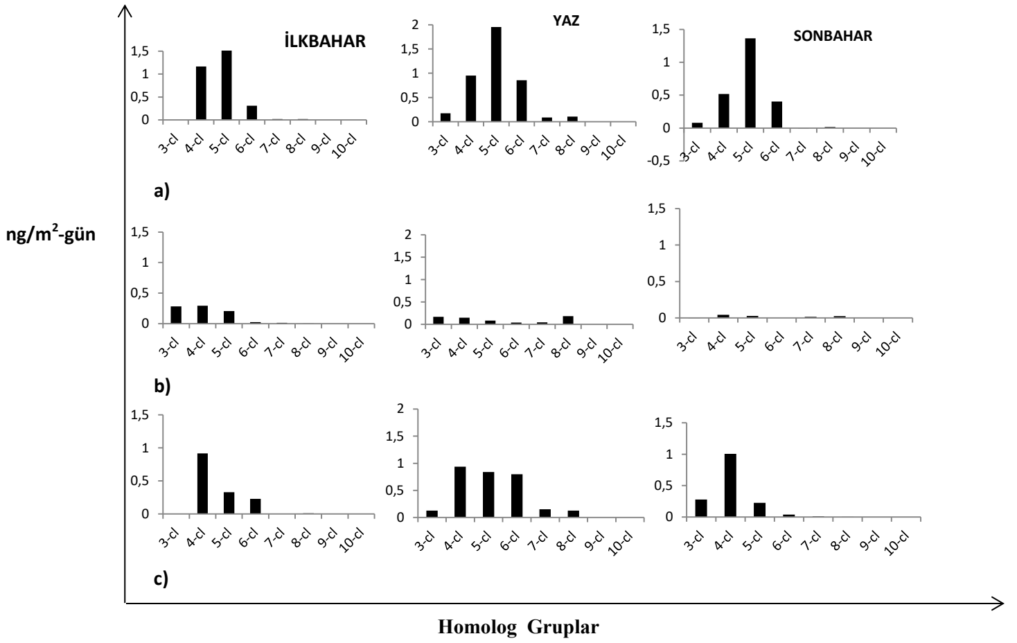
Şekil 4.17. Mevsimsel Fnet Homolog Grupları a)Endüstriyel b)Kentsel c)Yarı-Kırsal
