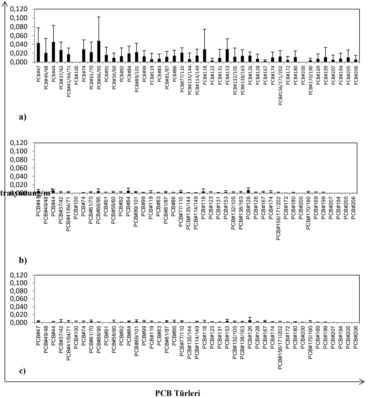
Şekil 4.14. Bursa'da Atmosferik Örneklerde PCB Konsantrasyonları a) Endüstriyel b) Kentsel c) Yarı-Kırsal
