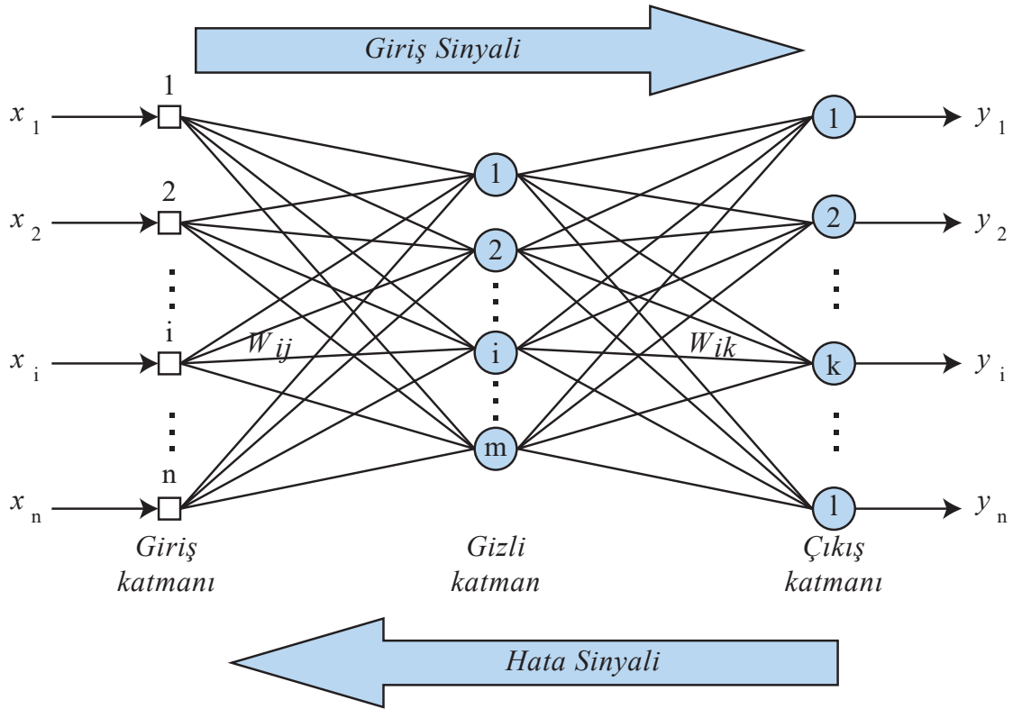
Şekil 2.5. Yapay sinir ağı yapısı 8
