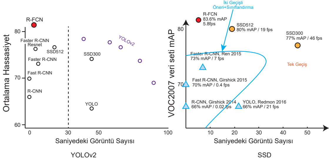
Şekil 3.2. R-CNN, YOLO ve SSD karşılaştırılması 16
