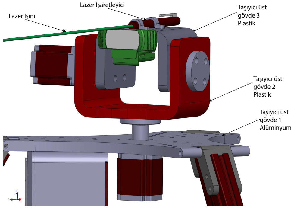
Şekil 3.16. Takip makinesi ebatlandırma görünüşü
