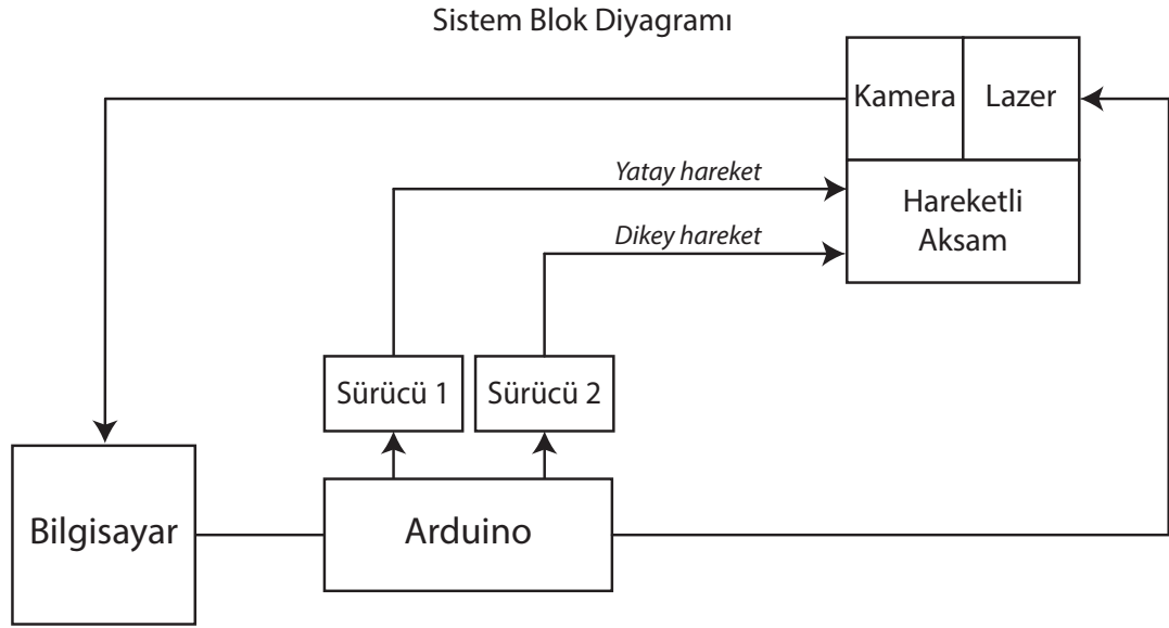
Şekil 3.13. Takip makinesi blok diyagramı
