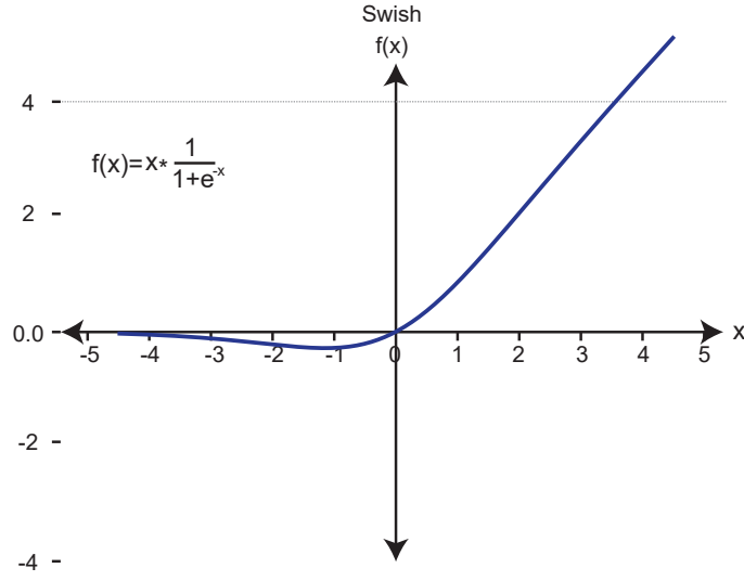
Şekil 2.9. Swish fonksiyonu
