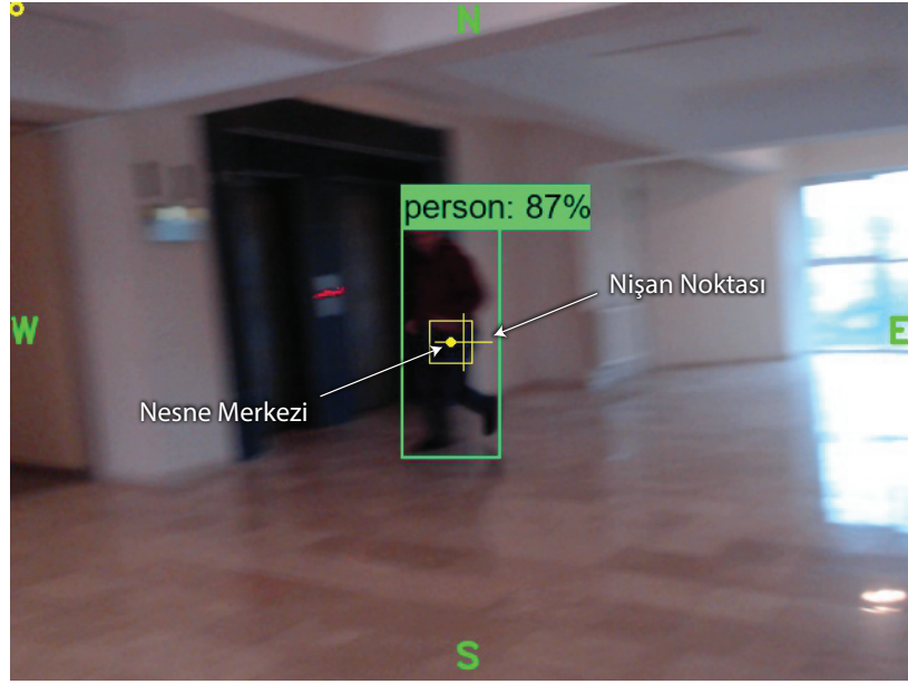
Şekil 4.7. İsbet görüntüsü, uzaklık=6,66 m, hız:10,34 km/saat
