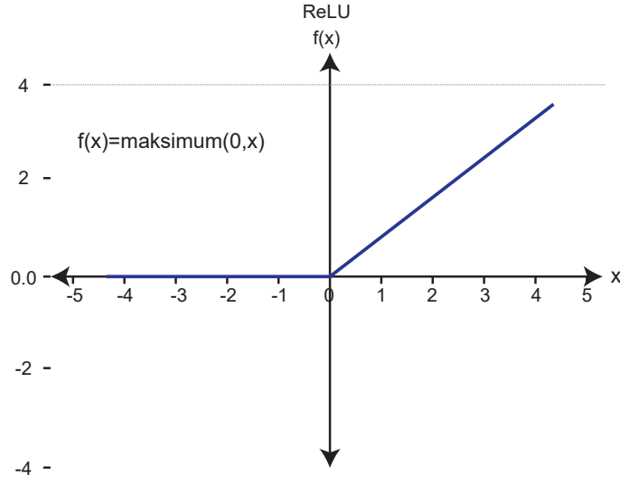
Şekil 2.6. ReLU
