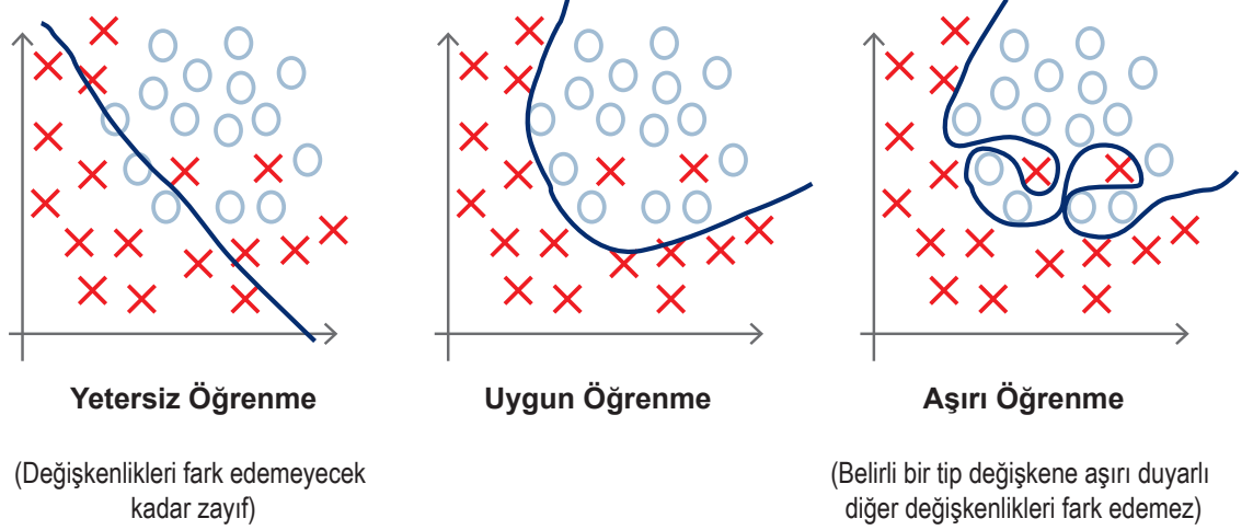
řekil 2.16. Ařırı ođrenme, Normal ođrenme ve Yetersiz ođrenme 12
