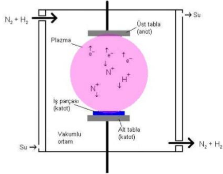
Şekil 2. 5. Plazma nitrüleme mekanizması (İğdil 2005)
