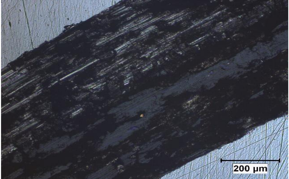
Şekil 4. 13. BM kodlu numunenin 0.7 kg yükte 15 mm/s kayma hızında oluşan aşınma optik mikroskop görüntüsü X100.
