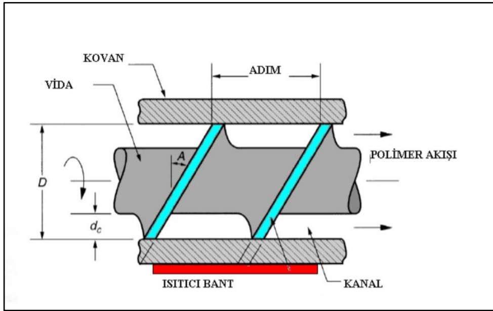
Şekil 3.2. Vida kovan sistemi
