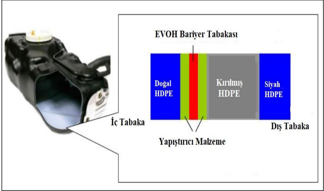
Şekil4.8. Çok katmanlı şekilde üretilen yakıt tankının kesiti
