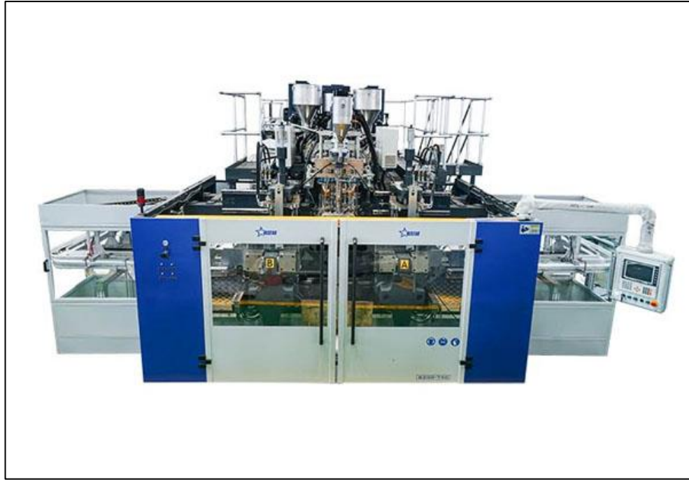
Şekil3.1. Şişirme makinesi
