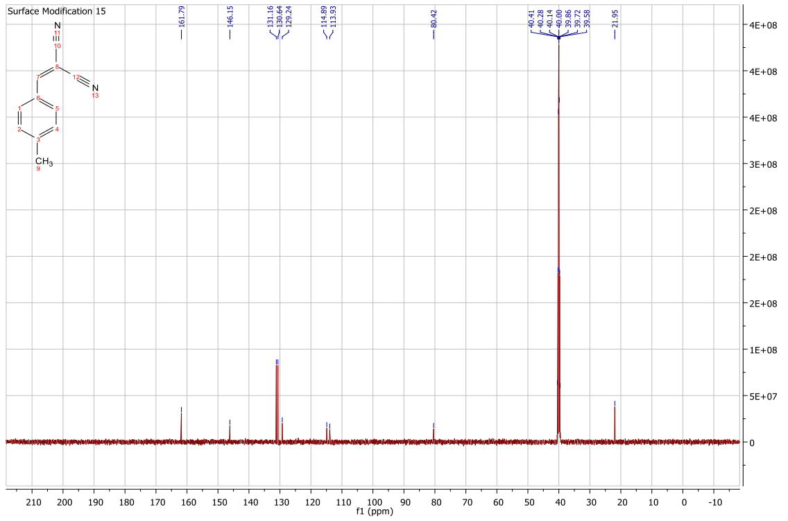
Ek 3.15. YM-15'in ^{13}\text{C} NMR spektrumu
