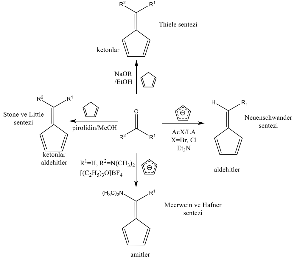
Şekil 2.17. Geleneksel Pentafulven sentezleri gösterimi
