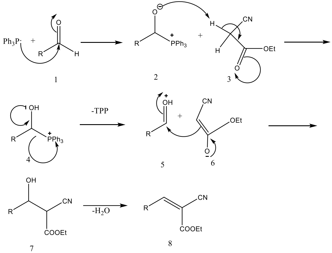
Şekil 2.5. TPP katalizörlüğünde gerçekleşen reaksiyonun mekanizması
