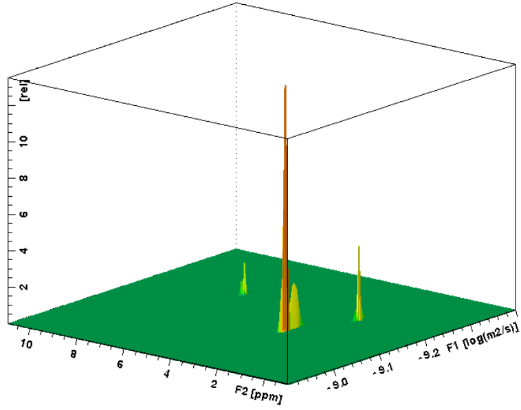
Şekil 4.14. Toluen bileşğinin DMSO-d 6 içerisindeki DOSY sonucu
