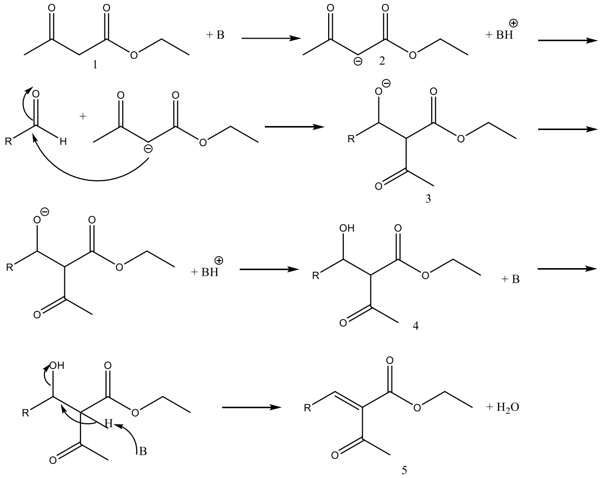
Şekil 2.2. Hann ve Lapworth Knoevenagel reaksiyon mekanizma önerisi
