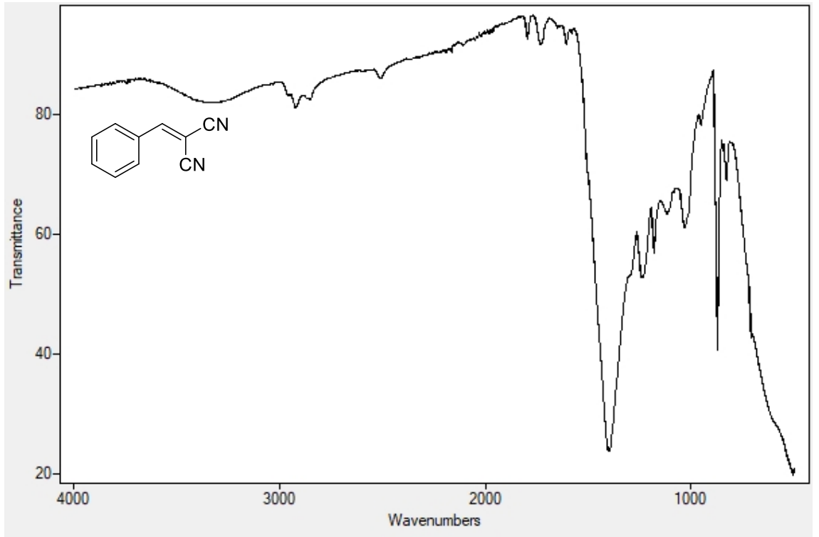
Ek 2.2. YM-11'in boya üzerinden FTIR spektrumu
