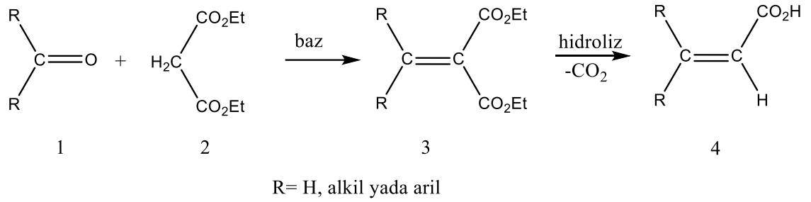
Şekil 2.1. Aldehit veya ketonlarla dietil malonatın kondenzasyon reaksiyonu
