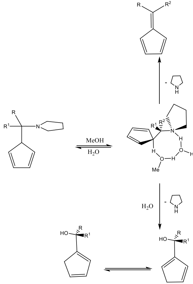
Şekil 2.20. Katalitik çevrimde çözücü etkisi
