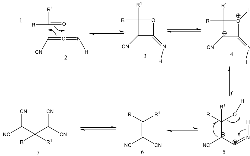
Şekil 2.11. Aprotik solvent içerisinde katalizörsüz Knoevenagel reaksiyonu
