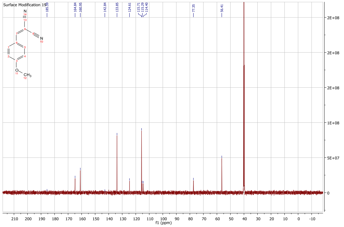
Ek 3.27. YM-19'un 13 C NMR spektrumu
