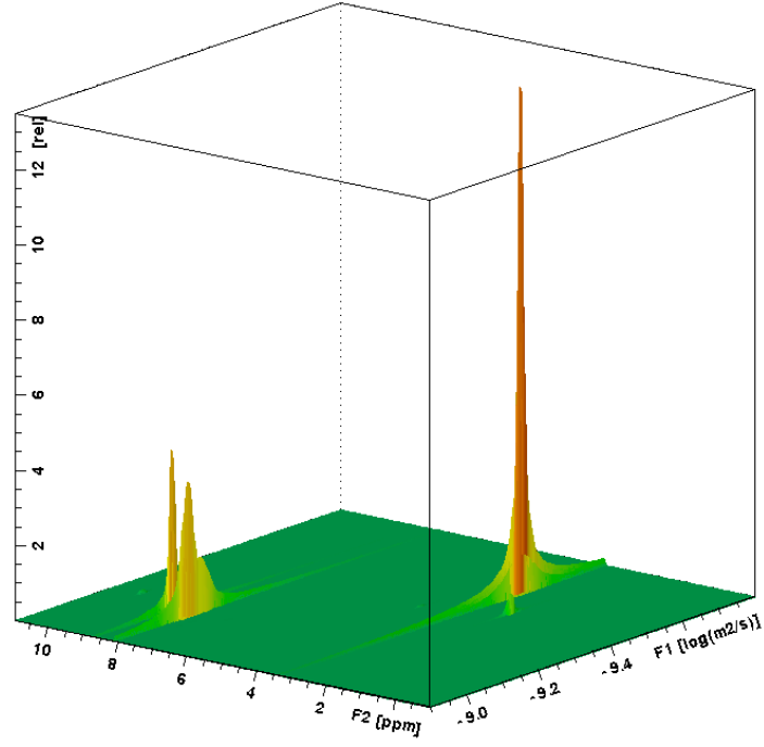
Şekil 4.13. YM-20 bileşğinin DMSO-d 6 içerisindeki DOSY sonucu
