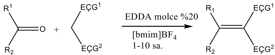
Şekil 2.7. İyonik sıvı içerisinde Knoevenagel kondenzasyonu
