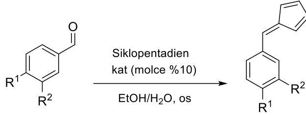
Şekil 3.3. Fulven sentezi genel gösterimi
