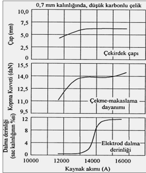
Şekil 2.8. Kaynak sırasında kaynak akımının çekirdek çapı, çekme dayanımı ve elektrod dalma derinliği üzerindeki etkileri (Kaya, 2010)
