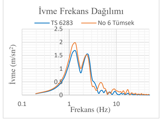
EK Şekil 3.13. V=40 km/sa için ivme-zaman ve frekans dağılımı
