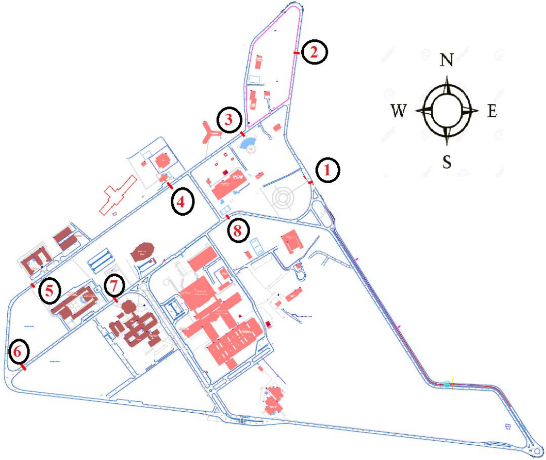
Şekil 3.1. BUÜ Görükle Kampüsü yol ağı ve çalışma için seçilen hız tümseklerinin konumları
