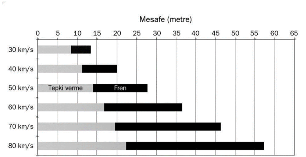
Şekil 2.1. Hızlara göre tepki verme frenleme mesafesi (WHO,2008)
