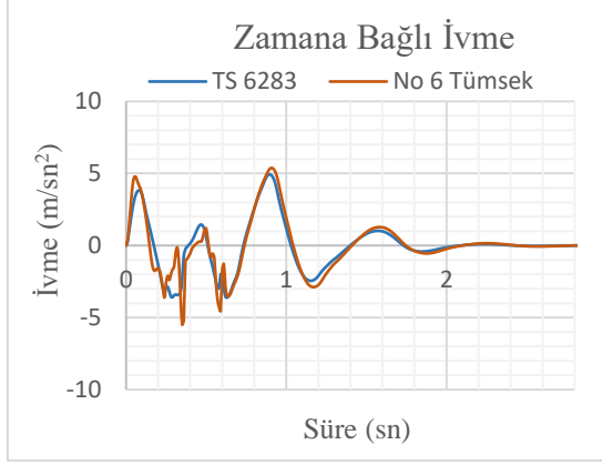
EK Şekil 3.13. V=40 km/sa için ivme-zaman ve frekans dağılımı
