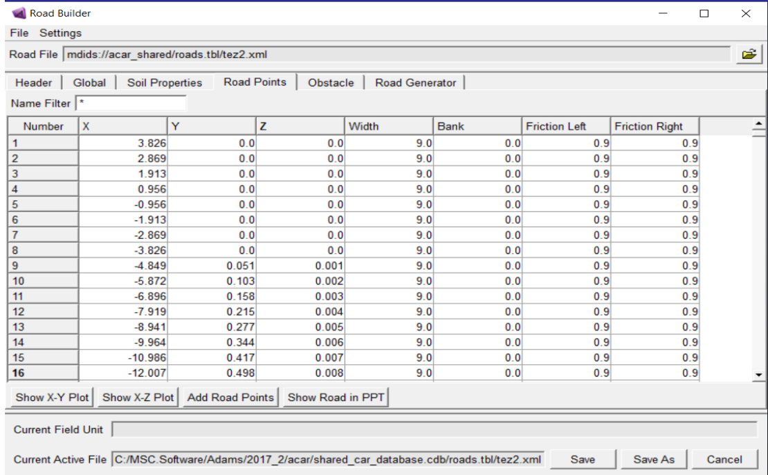
EK Şekil 4.1. Adams/Car ortamında üç boyutlu noktasal olarak yol oluşturma
