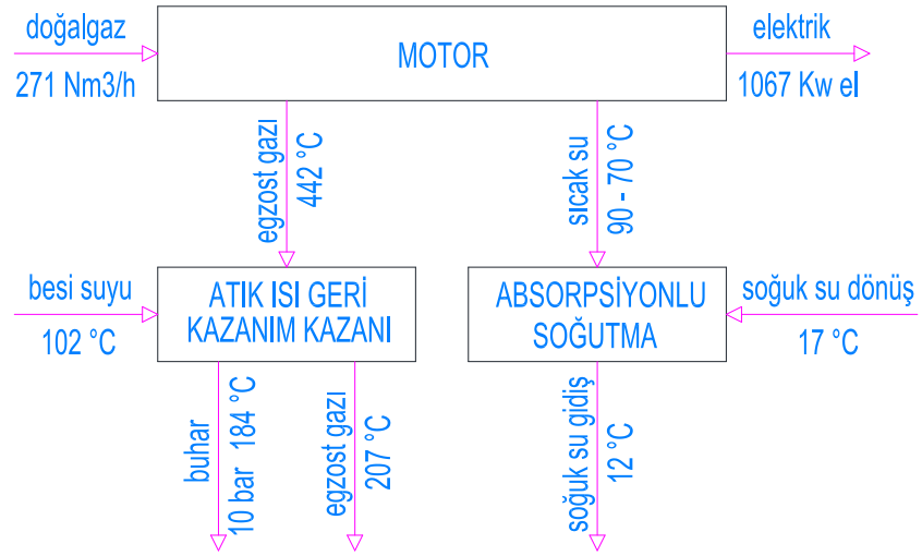
Şekil-13: Nominal Çalışma Durumu İçin Sistem Şeması
