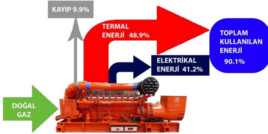
Şekil-4: Trijenerasyonun şematik görünüşü
