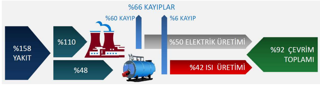
Şekil-3: Elektrik ve ısı enerjisinin ayrı ayrı üretilmesindeki verimler
