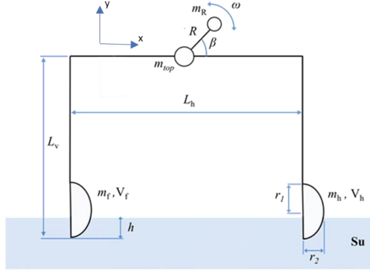
Şekil 3.3. Basitleştirilmiş sucul ilerleme modeli
