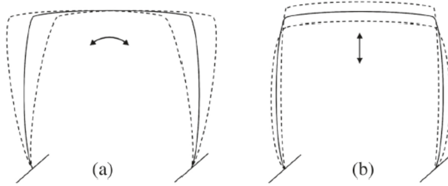
Şekil E.2.1. Elastik kirişin (a) burulma ve (b) boylamasına titreşimlerinin abartılı bir gösterimi
