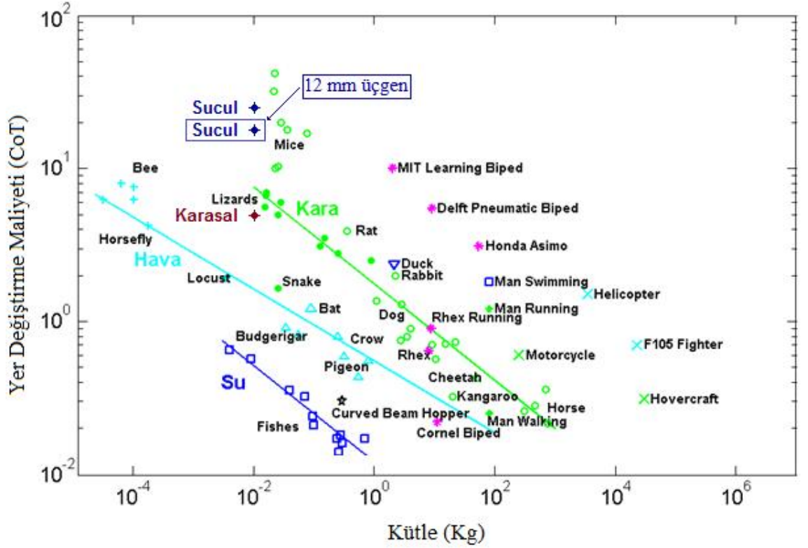
řekil 4.25. Mevcut mekanizmada 12 mm üçgen ayak kullanılması sonucu düşen sucul yer deęiřtirme maliyetinin Tucker diyagramında gösterimi
