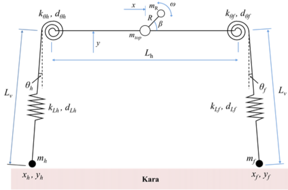
Şekil 3.2. Basitleştirilmiş karasal ilerleme modeli
