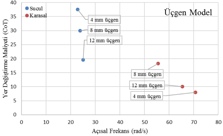
Őekil 4.23. Üçgen model ayak yapıları için sucul ve karasal ilerlemelerde en düşük yer deęiřtirme maliyet deęerleri
